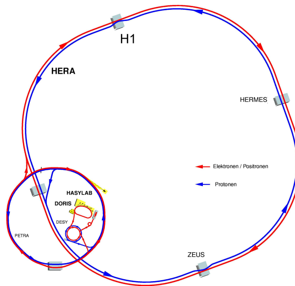
Abbildung 2.1: Der Elektron-Proton-Speicherring HERA mit seinen Vorbeschleunigern
