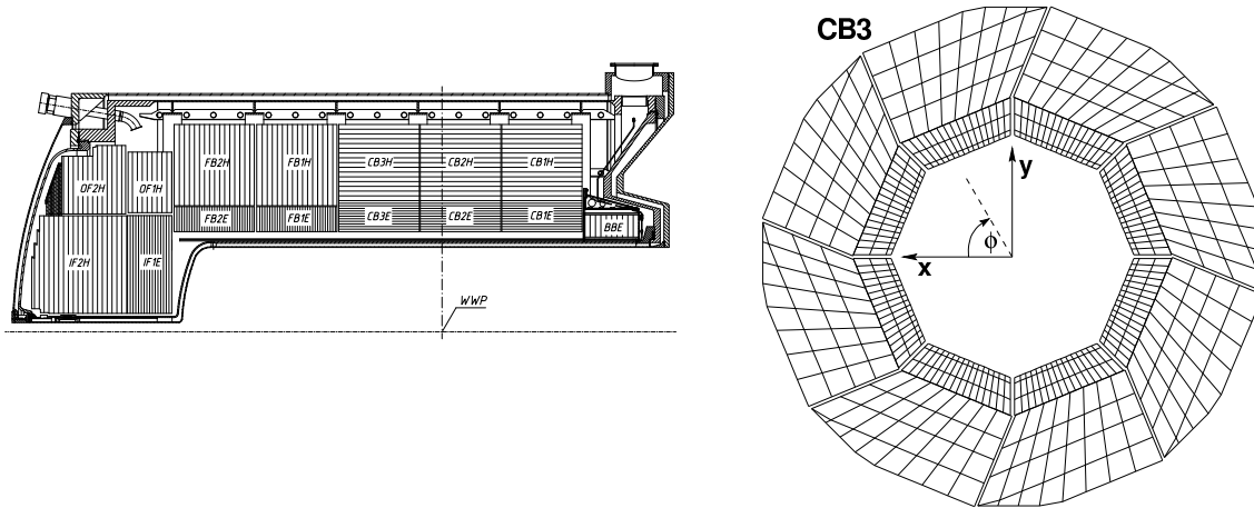
Abbildung 2.4: Flüssig-Argon-Kalorimeter, links ist das LAr-Kalorimeter im Längsschnitt dargestellt. Zu erkennen ist der Aufbau aus Rädern sowie die unterschiedliche Ausrichtung der Lagen. Rechts ist ein einzelnes Rad in der xy -Ebene dargestellt. Hier werden die Lücken zwischen den Oktanten sichtbar.
