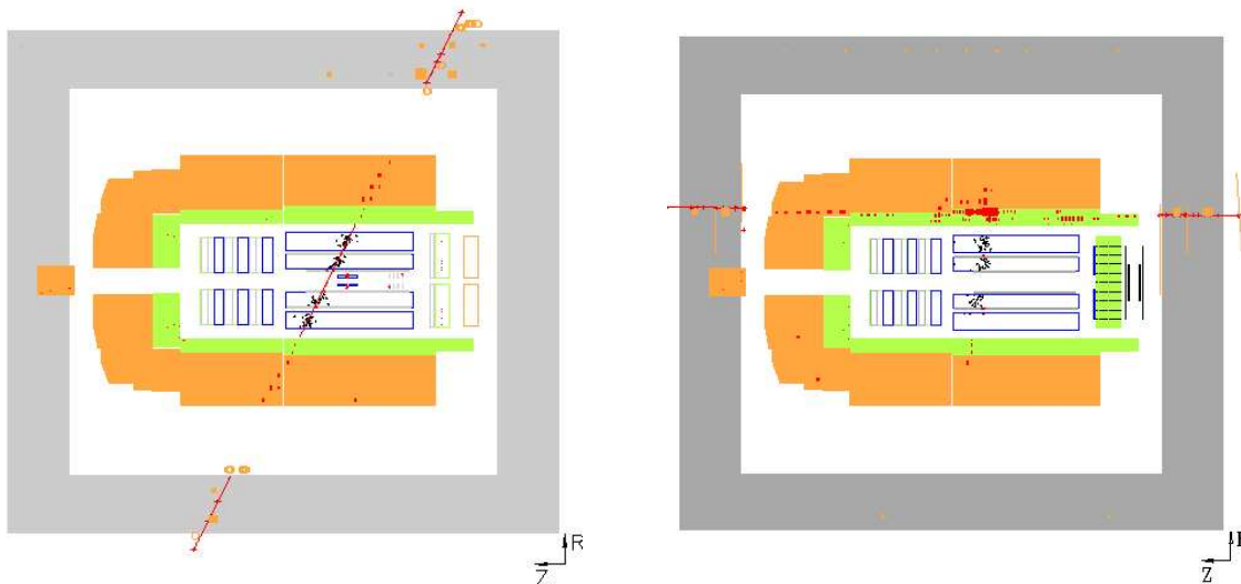
Abbildung 3.2: Links ist eine graphische Ereignisdarstellung zu sehen, die ein Myon aus der kosmischen Höhenstrahlung zeigt. Rechts ist ein Ereignis mit einem Halomyon dargestellt.
