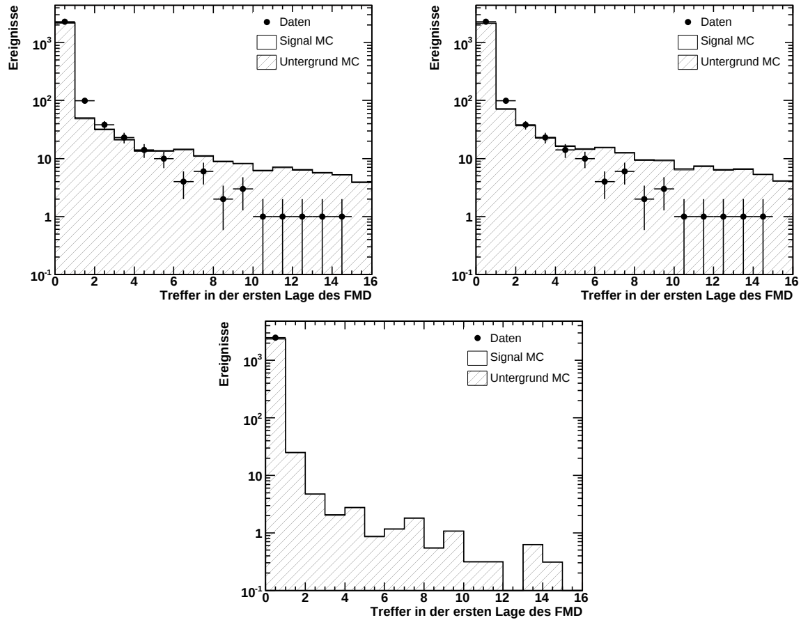
Abbildung 4.19: Simulation des Rauschens im Vorwärts-Myonsystem. Es sind jeweils die Treffer der ersten Lage des Vorwärts-Myonsystems aufgetragen. Oben links ist die Verteilung der Treffer ohne die zusätzliche Simulation des Rauschens dargestellt, oben rechts mit dieser. Unten ist die Verteilung des reinen simulierten Rauschens zu sehen.
