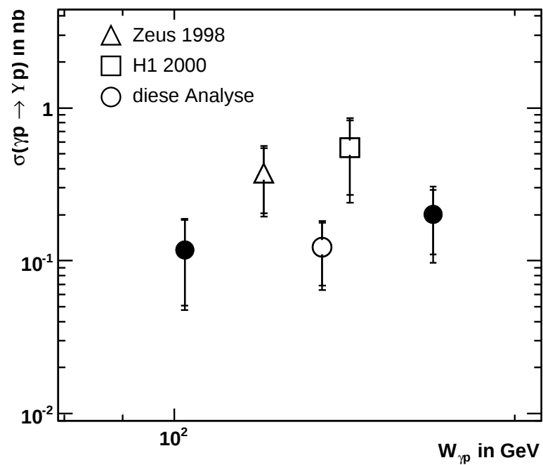
Abbildung 5.26: \gamma p -Wirkungsquerschnitt als Funktion von W_{\gamma p} . Dargestellt durch die Kreise sind die Ergebnisse dieser Analyse. Der offene Kreis berücksichtigt den gesamten W_{\gamma p} -Bereich, die gefüllten Kreise zeigen die Ergebnisse der W_{\gamma p} -Teilbereiche. Zum Vergleich sind die Ergebnisse der Veröffentlichungen von Zeus [Bre98b] und H1 [Adl00] dargestellt.
