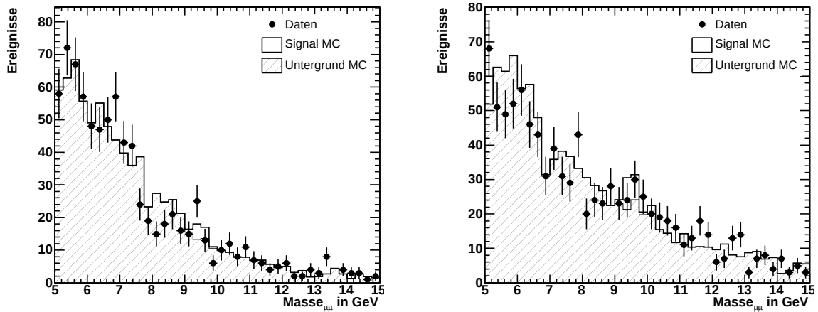
Abbildung 4.26: Massenverteilung nach allen Schnitten. Links ist die Massenverteilung des ersten W_{\gamma p} -Bereiches W_{gp1} = [70 \text{ GeV}, 115 \text{ GeV}] zu sehen, rechts der entsprechende zweite Bereich mit W_{gp2} = [115 \text{ GeV}, 250 \text{ GeV}] .
