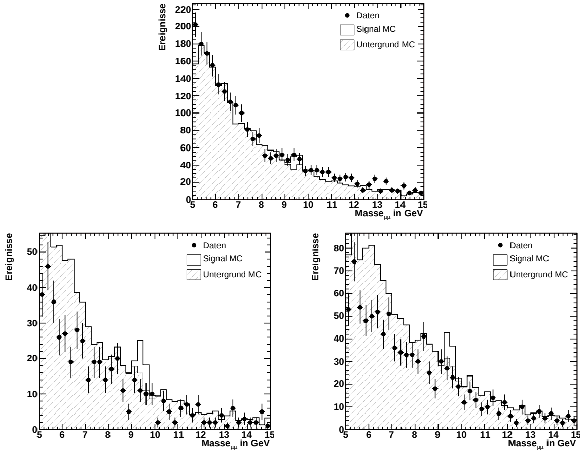
Abbildung 4.21: Im oberen Histogramm ist die Verteilung der invarianten Masse mit den Schnitten für elastische \gamma zu sehen. Unten links sind diejenigen Ereignisse dargestellt, die durch die Bedingungen der Vorwärtsdetektoren verworfen werden. Unten rechts sind ebenfalls die verworfenen Ereignisse zu sehen, wobei zusätzlich die Forderung für den Impulsübertrag am Protonvertex auf -t < 10 \text{ GeV}^2 gelockert worden ist.
