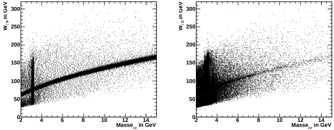
Abbildung 4.4: Photon-Proton-Schwerpunktsenergie gegen die invariante Masse des Spurpaars. Links ist diese Verteilung vor Berücksichtigung des J/\Psi -Untergrundindikators zu sehen, rechts mit der Forderung, daß dieser nicht gesetzt worden ist.
