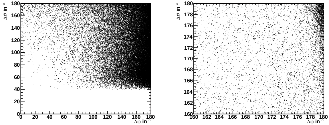
Abbildung 4.6: Öffnungswinkel \Delta\vartheta und \Delta\varphi der beiden Myonkandidaten nach den bisher angewandten kosmischen Schnitten.
