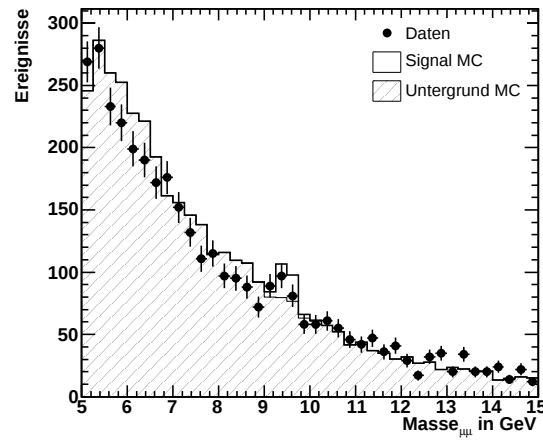
Abbildung 4.14: Verteilung der invarianten Masse mit der Bedingung, nur zwei Lee-West-Spuren gefunden zu haben.
