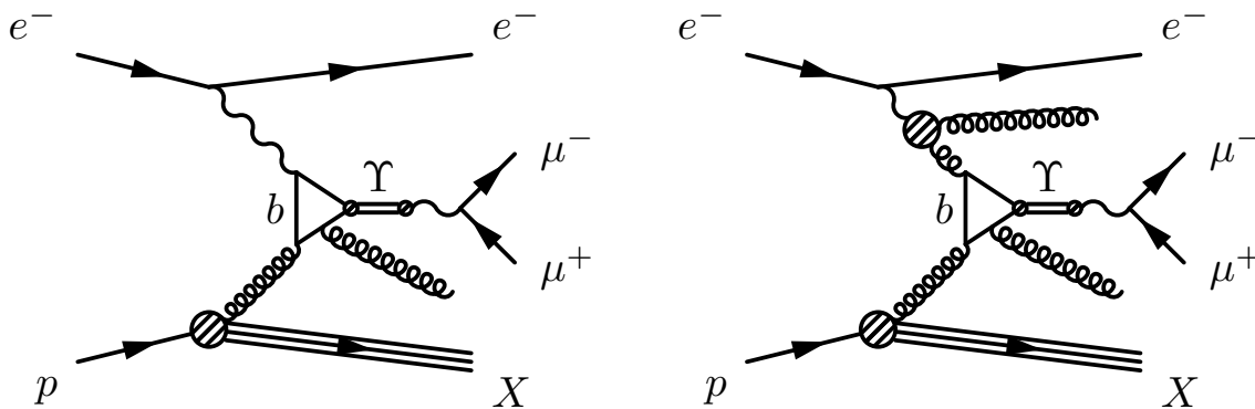
Abbildung 1.4: Im linken Feynmandiagramm sieht man die direkte Photon-Gluon-Fusion zur Erzeugung eines \Upsilon -Mesons. Rechts ist die Gluon-Gluon-Fusion, der Prozeß mit aufgelöstem Photon, zu sehen.
