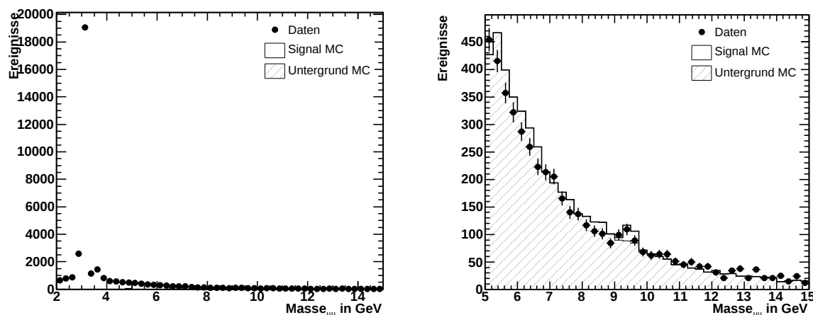
Abbildung 4.9: Massenverteilung nach der Forderung, zwei Myonen mit den oben beschriebenen Qualitätsanforderungen identifiziert zu haben.
