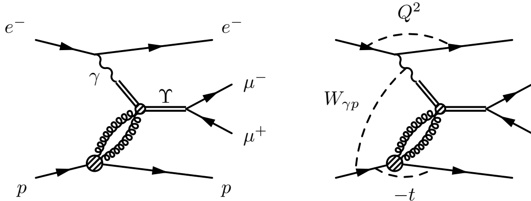
Abbildung 4.15: Im linken Graphen ist nochmals die diffraktive \Upsilon -Produktion dargestellt mit dem anschließenden Zerfall in zwei Myonen. Rechts sieht man die zugehörigen kinematischen Variablen, den Impulsübertrag des Elektrons Q^2 , des Protons -t sowie die Photon-Proton-Schwerpunktsenergie W_{\gamma p} .
