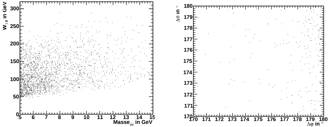
Abbildung 4.24: Kontrollverteilungen für kosmische Myonen nach dem Schnitt auf den Ereigniszeitpunkt. Links ist W_{\gamma p} gegen die invariante Masse gezeigt, rechts \Delta\vartheta gegen \Delta\varphi .
