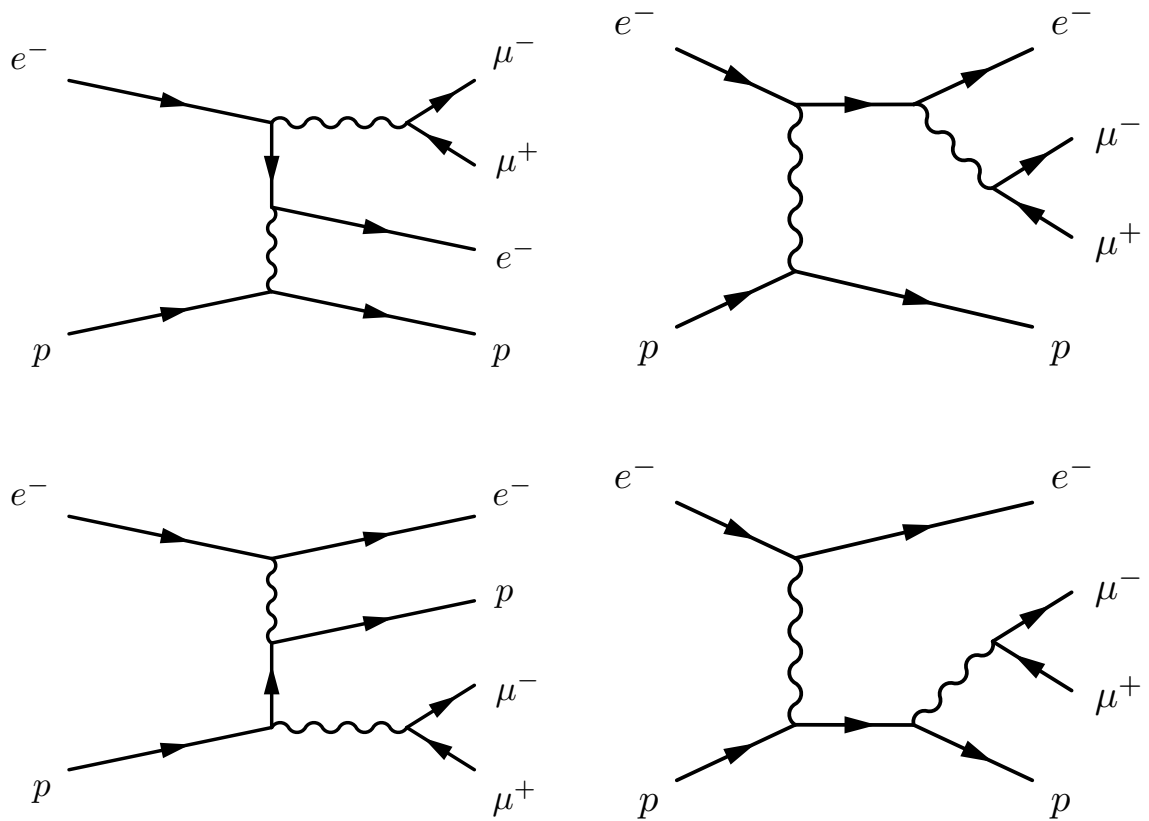
Abbildung 1.6: Hier sind die Produktionsprozesse zu sehen, bei denen ein Photon der Bremsstrahlung in ein Myonpaar konvertiert. In der oberen Reihe stammt das Photon vom Elektron, wohingegen in der unteren Reihe das Proton das Photon emittiert. Links sind die Prozesse mit Ausstrahlung des Photons im Anfangszustand dargestellt, rechts wird das Photon im Endzustand ausgesandt.
