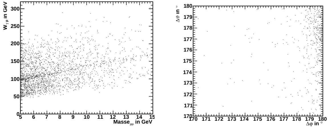
Abbildung 4.22: Kontrollverteilungen für kosmische Myonen nach den Schnitten für die elastische Selektion. Links ist W_{\gamma p} gegen die invariante Masse gezeigt, rechts ist \Delta\varphi gegen \Delta\vartheta dargestellt.
