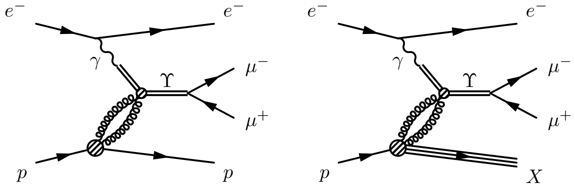
Abbildung 1.3: Feynmangraphen der diffraktiven \Upsilon -Produktion in niedrigster Ordnung. Links ist der elastische Prozeß zu sehen, rechts der Prozeß, bei dem das Proton dissoziiert. Das vom Elektron abgestrahlte Photon fluktuiert in ein b\bar{b} -Paar und wird durch den Austausch zweier Gluonen auf die Massenschale des \Upsilon gehoben. Der Gluonenaustausch erfolgt in diffraktiven Prozessen so, daß das b\bar{b} -Paar ein farbneutrales System bildet.
