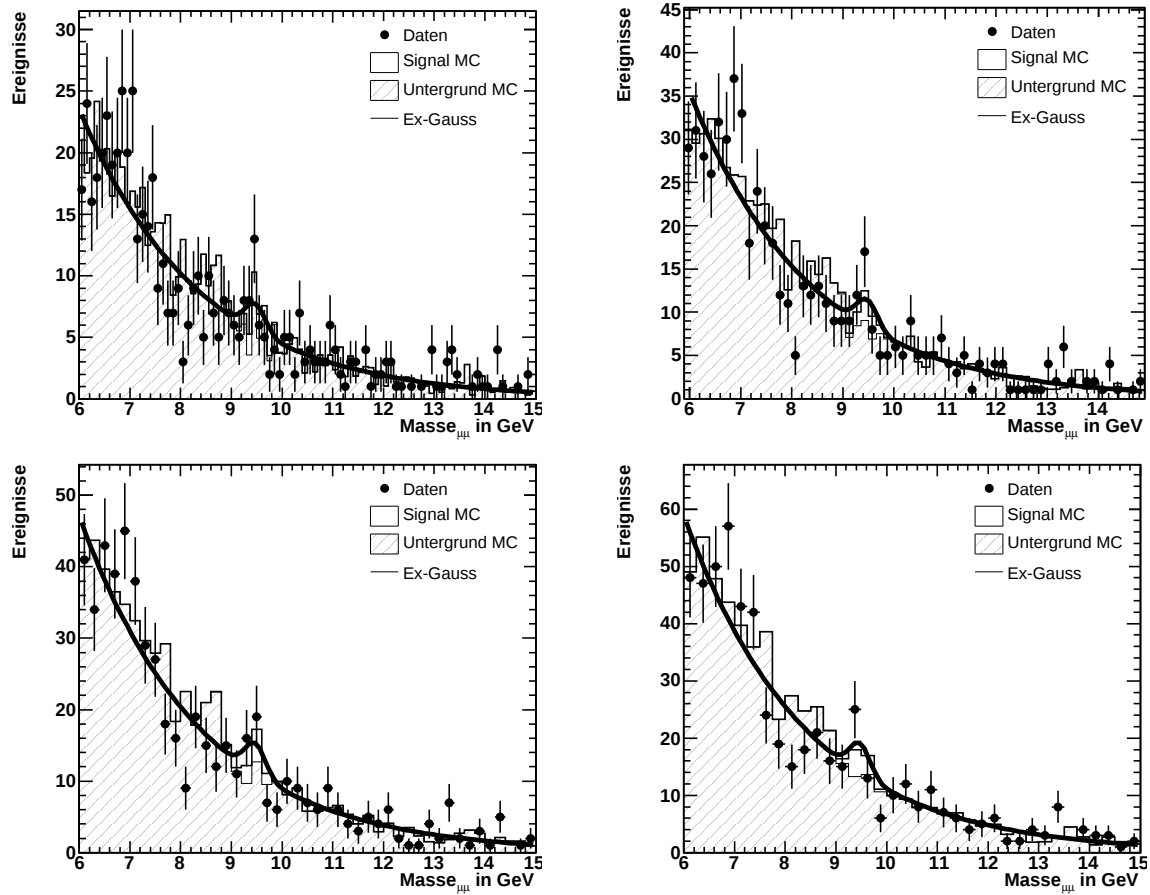
Abbildung 5.6: Anpassung der Daten im Bereich Wgp1 durch die Summe einer Exponential- und einer Gaußfunktion. Dabei wurden die Energieabhängigkeit des Untergrundes, die Resonanzmasse und -breite durch die Werte der MonteCarlo-Simulation fixiert. Die Histogramme zeigen die Anpassungen mit den Binbreiten [100, 150, 200, 250] in MeV. Die Ergebnisse sind in Tabelle 5.4 dargestellt.
