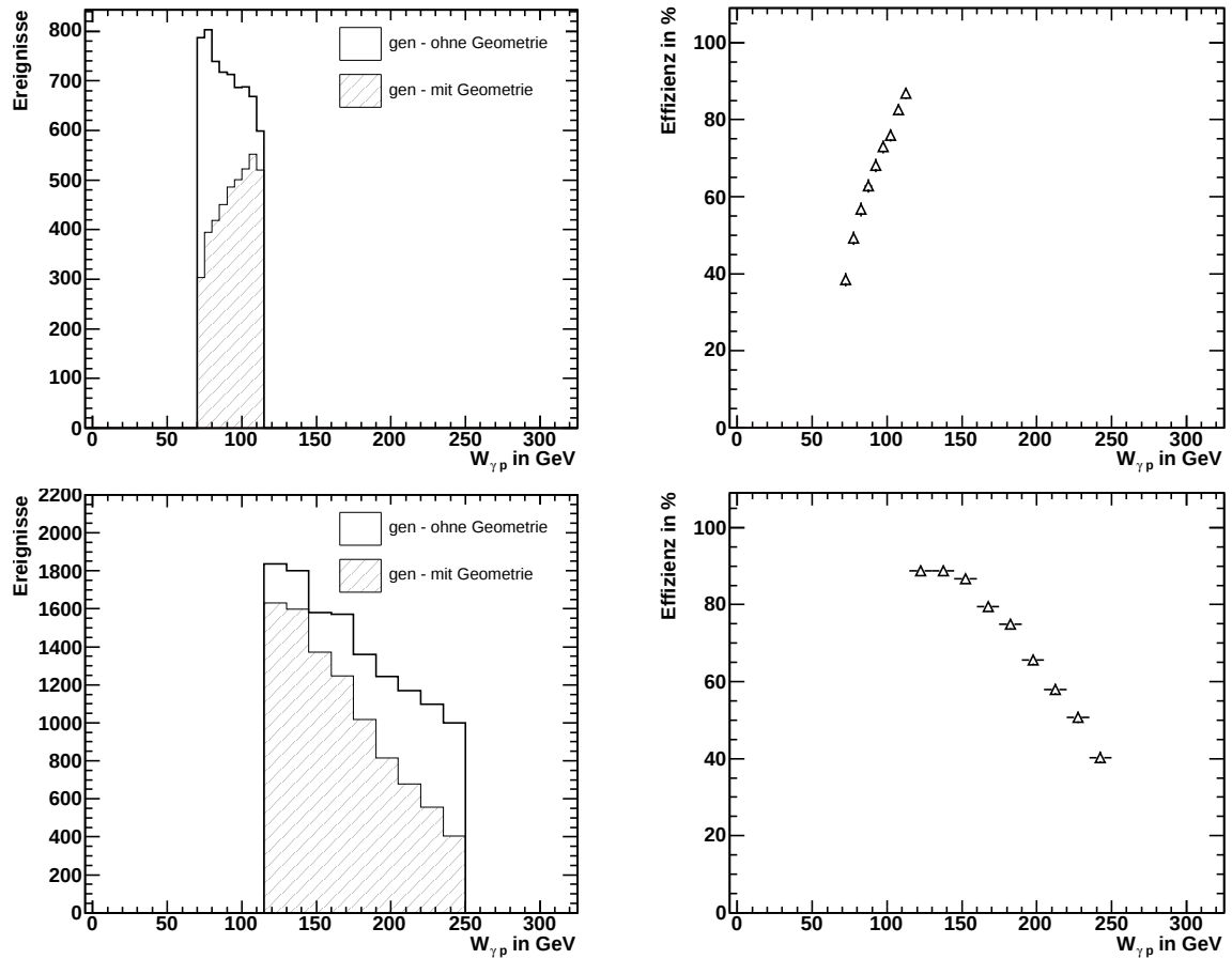
Abbildung 5.15: Geometrische Akzeptanz. Oben ist die Akzeptanz für den ersten W_{\gamma p} -Bereich von 70 GeV bis 115 GeV dargestellt, unten für den Bereich von 115 GeV bis 250 GeV.
