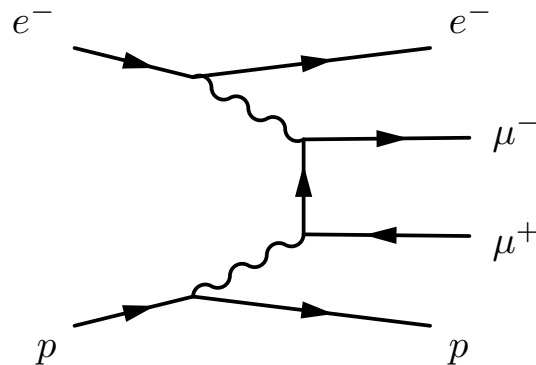
Abbildung 3.1: Dieser reine QED Feynmangraph zeigt den wichtigsten Untergrundprozeß, die Myonpaar-Photoproduktion.
