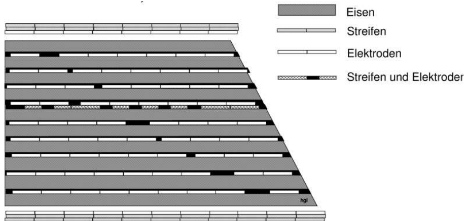
Abbildung 2.6: Anordnung der sensitiven Lagen im zentralen Myondetektor
