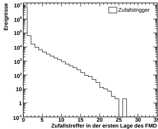
Abbildung 4.18: Anzahl der Treffer in der ersten Lage des Vorwärts-Myonsystems, die mit dem Zufallstrigger aufgezeichnet wurden.
