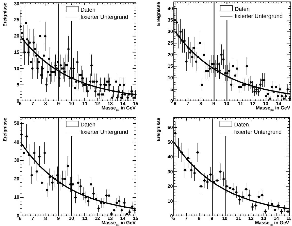
Abbildung 5.9: Ereigniszahlen für den Bereich Wp2. Es wird die Differenz aus Untergrund- erwartung und der Anzahl der gemessenen Datenereignisse innerhalb des durch die Geraden gekennzeichneten Bereichs [9.0 GeV - 10.0 GeV] summiert. Die Ergebnisse stehen in Tabelle 5.5.
