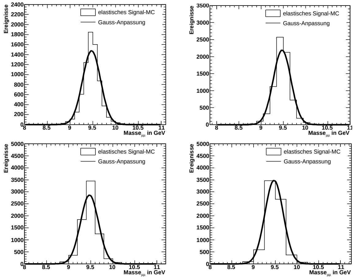
Abbildung 5.1: Anpassung der Massenverteilung der elastischen Signal-MonteCarlo-Simulation durch eine Gaußkurve. Die einzelnen Histogramme zeigen die Anpassung mit der Variation der Binbreiten. Diese variieren von oben links von 100 MeV über 150 MeV und 200 MeV bis 250 MeV unten rechts. Die Ergebnisse der Anpassungen sind in Tabelle 5.1 dargestellt.
