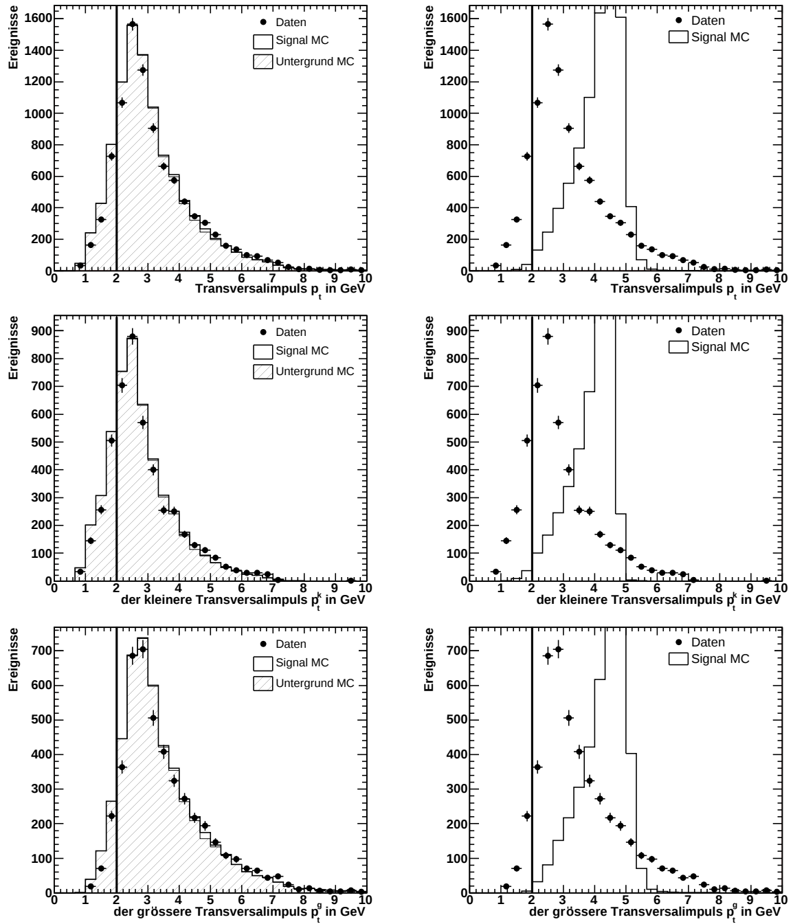
Abbildung 4.10: In den Abbildungen ist der Transversalimpuls der Myonen zu sehen. Links sind die Daten mit den Untergrund- und Signal-MonteCarlo-Simulationen dargestellt. Rechts sind die Daten nur mit der auf die Datenereigniszahl normierten Signal-MonteCarlo-Simulation gezeigt. In den Histogrammen der obersten Zeile sind alle Transversalimpulse, in der zweiten Zeile ist nur der jeweils kleinere und in der dritten Zeile der jeweils größere Transversalimpuls der beiden Myonen eingetragen. Die Forderung von p_t \geq 2.0 GeV wurde in alle Abbildungen eingezeichnet.
