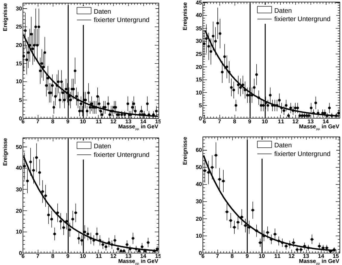
Abbildung 5.8: Ereigniszahlen für den Bereich W_{p1} . Es wird die Differenz aus Untergrund- erwartung und der Anzahl der gemessenen Datenereignisse innerhalb des durch die Geraden gekennzeichneten Bereichs [9.0 \text{ GeV} - 10.0 \text{ GeV}] summiert. Die Ergebnisse stehen in Tabelle 5.5.
