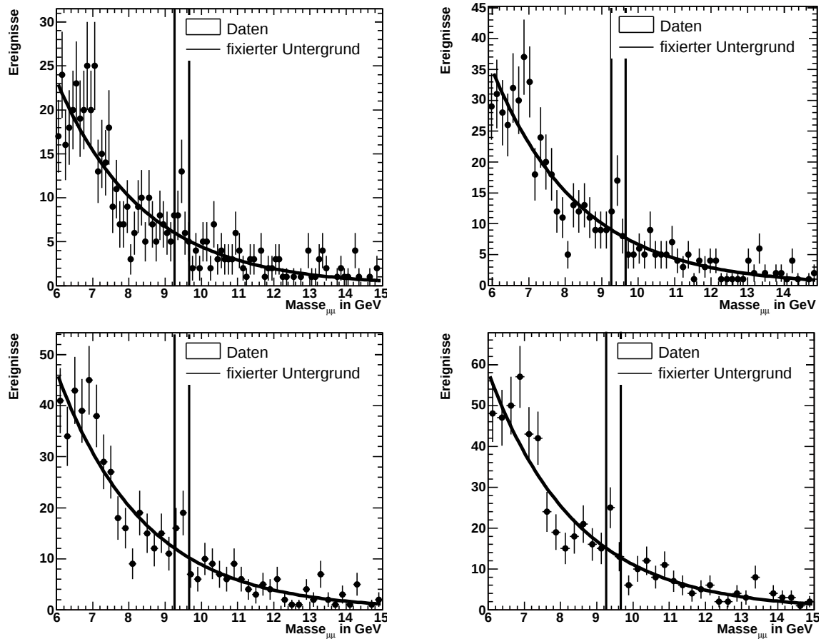
Abbildung 5.10: Ereigniszahlen für den Bereich Wgp1. Es wird die Differenz aus Untergrunderwartung und der Anzahl der gemessenen Datenereignisse innerhalb des durch die Geraden gekennzeichneten Bereichs [9.26 \text{ GeV} - 9.66 \text{ GeV}] summiert. Die Ergebnisse stehen in Tabelle 5.6.
