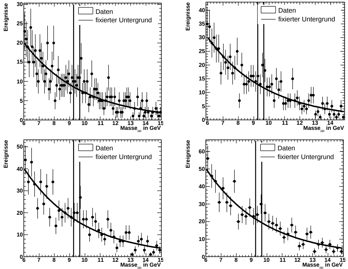
Abbildung 5.11: Ereigniszahlen für den Bereich Wgp2. Es wird die Differenz aus Untergrunderwartung und der Anzahl der gemessenen Datenereignisse innerhalb des durch die Geraden gekennzeichneten Bereichs [9.26 GeV - 9.66 GeV] summiert. Die Ergebnisse stehen in Tabelle 5.6.
