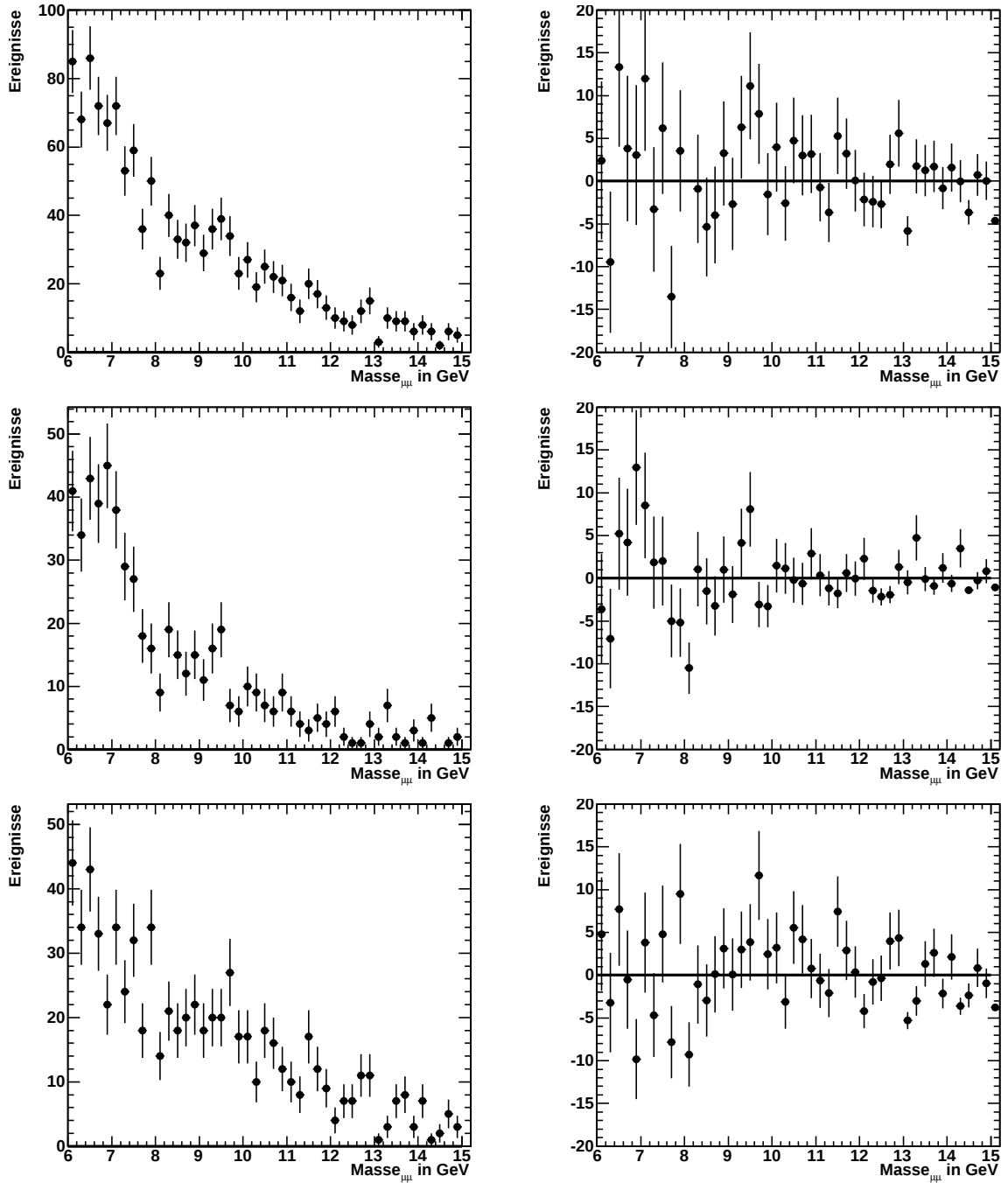
Abbildung 5.12: Verteilung der invarianten Masse des Datensatzes und Differenz zur Untergrunderwartung. In der obersten Zeile ist die Verteilung für den gesamten W_{\gamma p} -Bereich von 70 GeV bis 250 GeV zu sehen, in der mittleren Zeile für W_{\gamma p1} und in der letzten für W_{\gamma p2} . Rechts ist die Differenz der Datenverteilung und der Untergrunderwartung zu sehen, wie sie aus der Anpassung mit fünf freien Parametern gewonnen wurde. Die Binbreite beträgt 200 MeV.
