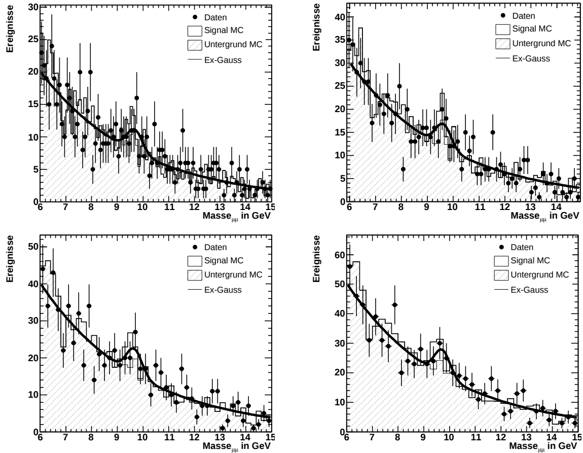
Abbildung 5.5: Anpassung der Daten im Bereich W_{p2} durch die Summe einer Exponential- und einer Gaußfunktion. Die Histogramme zeigen die Anpassungen mit den Binbreiten [100, 150, 200, 250] in MeV. Die Ergebnisse sind in Tabelle 5.3 zu sehen.
