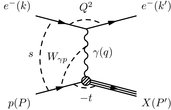
Abbildung 1.1: Feynmangraph der ep -Streuung in niedrigster Ordnung.
