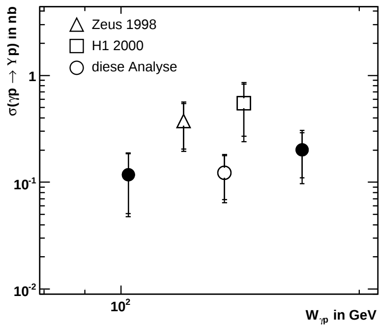
Abbildung 6.1: \gamma p -Wirkungsquerschnitt als Funktion von W_{\gamma p} . Dargestellt durch die Kreise sind die Ergebnisse dieser Analyse. Der offene Kreis berücksichtigt den gesamten W_{\gamma p} -Bereich, die gefüllten Kreise zeigen die Ergebnisse der W_{\gamma p} -Teilbereiche. Zum Vergleich sind die Ergebnisse der Veröffentlichungen von Zeus [Bre98b] und H1 [Adl00] dargestellt.
