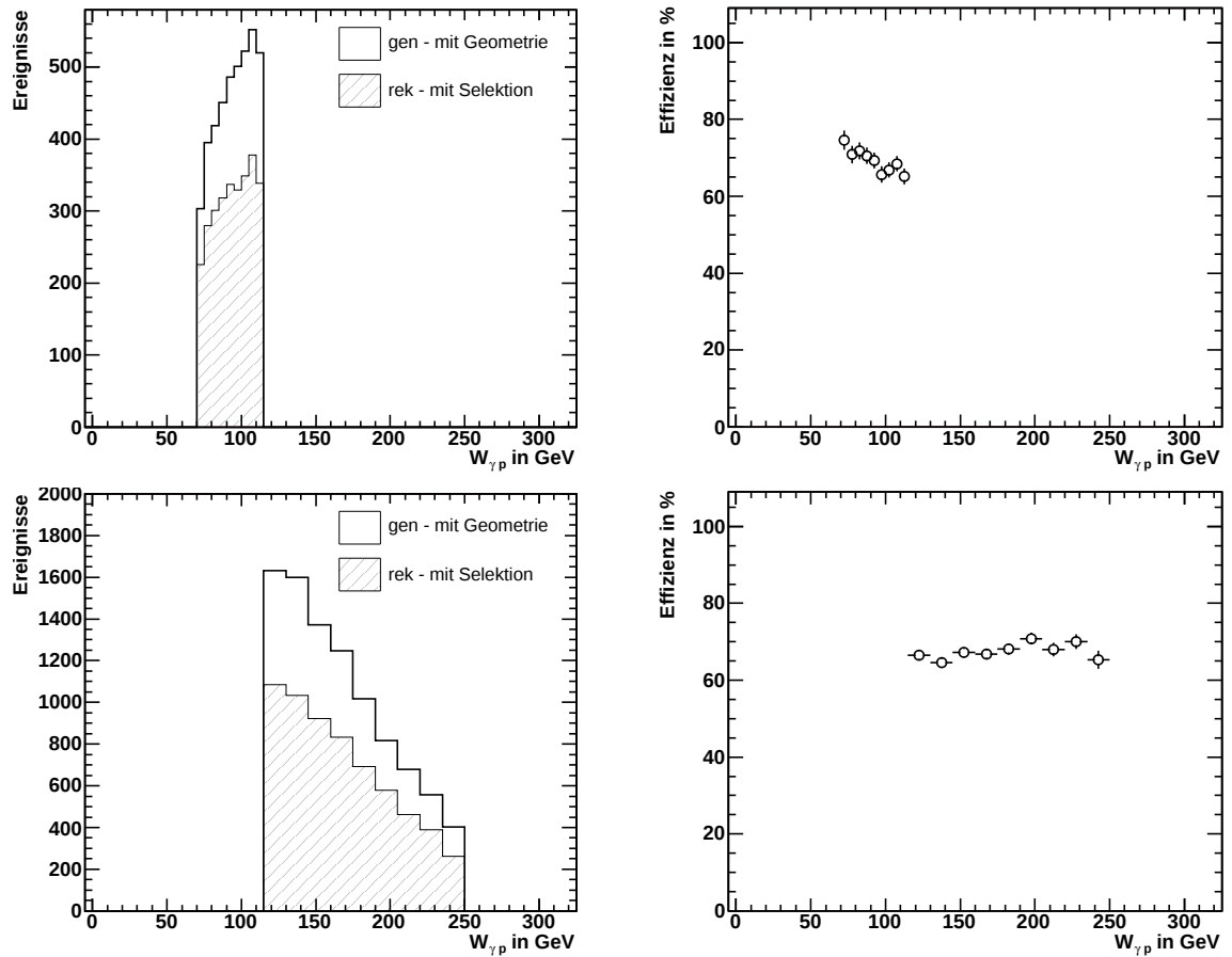
Abbildung 5.17: Selektionseffizienz. Oben ist die Selektionseffizienz für den ersten W_{\gamma p} -Bereich von 70 GeV bis 115 GeV dargestellt, unten für den Bereich von 115 GeV bis 250 GeV.
