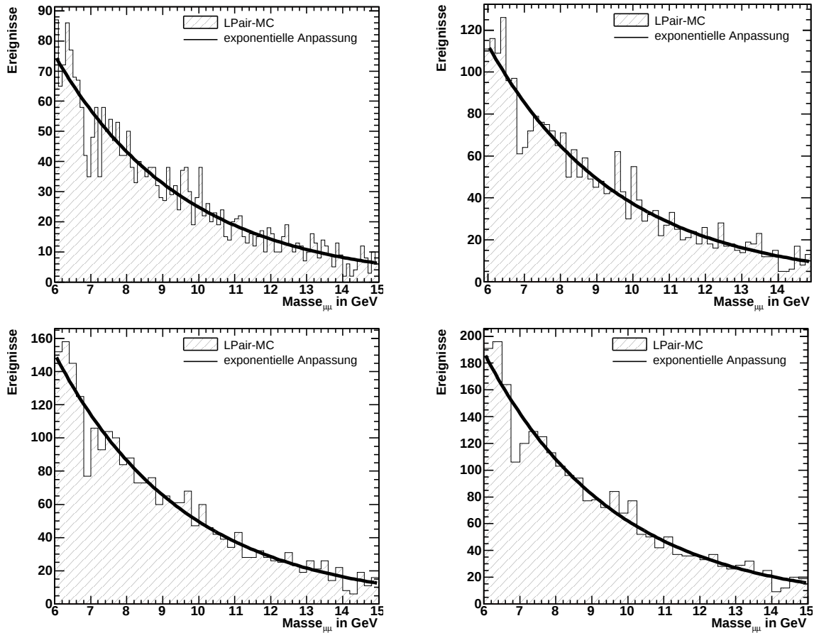
Abbildung 5.3: Anpassung des Untergrundes im Bereich W_{gp2} , der durch den MonteCarlo-Generator LPair erzeugt wird, mittels einer Exponentialfunktion. Die Histogramme zeigen die Anpassung mit den Binbreiten [100, 150, 200, 250] in MeV. Die Ergebnisse sind in Tabelle 5.2 zu sehen.
