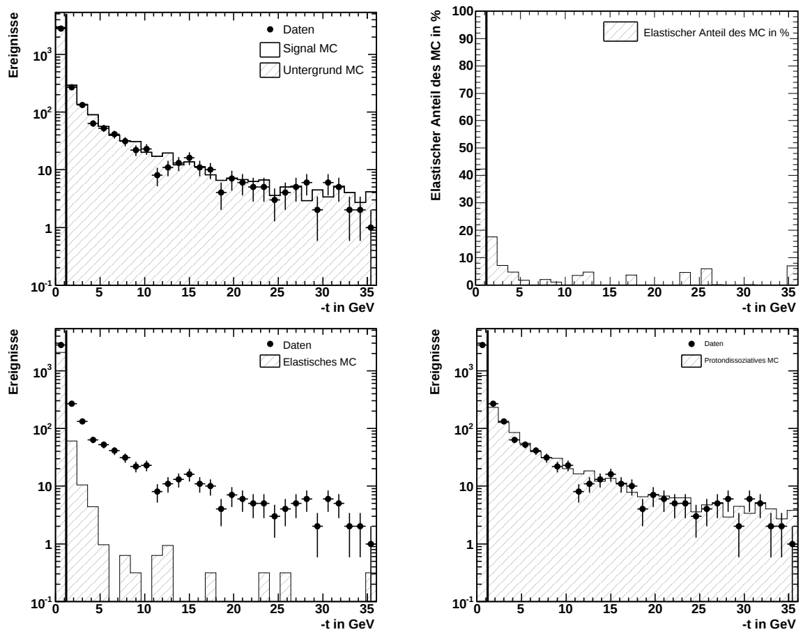
Abbildung 4.16: Verteilung des Impulsübertrages -t am Protonvertex. Eingezeichnet ist auch der Schnitt bei 1.2 GeV, der alle Ereignisse mit größerem Übertrag verwirft. Links oben sind die Daten mit der gesamten MonteCarlo-Erwartung zu sehen. Unten ist diese Erwartung in den elastischen (links) und protodissoziativen Anteil (rechts) unterteilt. Oben rechts ist der Anteil der elastischen an der gesamten MonteCarlo-Erwartung für jedes Intervall in Prozent zu sehen.
