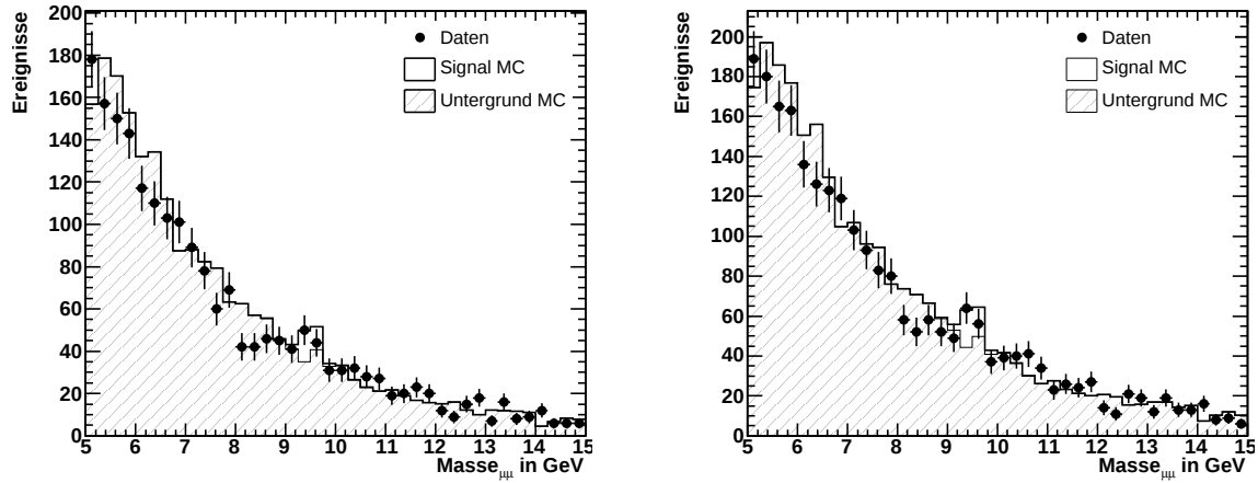
Abbildung 4.25: Links: Verteilung der invarianten Masse nach allen Schnitten. Rechts: Verteilung der invarianten Masse nach allen Schnitten, bis auf die Schnitte auf die Impulsüberträge an den Vertices ( Q^2 und -t ).
