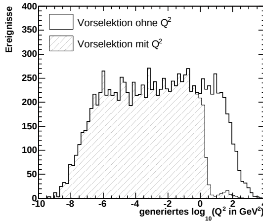
Abbildung 4.2: Generierte Verteilung von Q^2 aus der elastischen Signal-MonteCarlo-Simulation. Das leere Histogramm zeigt die Verteilung mit den Schnitten der Vorselektion, jedoch ohne den Q_e^2 -Schnitt, schraffiert ist die Verteilung mit dem Q_e^2 -Schnitt gezeigt.
