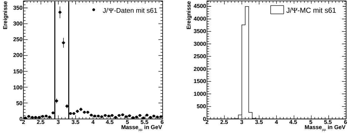
Abbildung 5.18: Massenverteilung des J/\Psi mit s61. Links sind die Daten zu sehen, rechts die MonteCarlo-Simulation für tiefunelastische J/\Psi .
