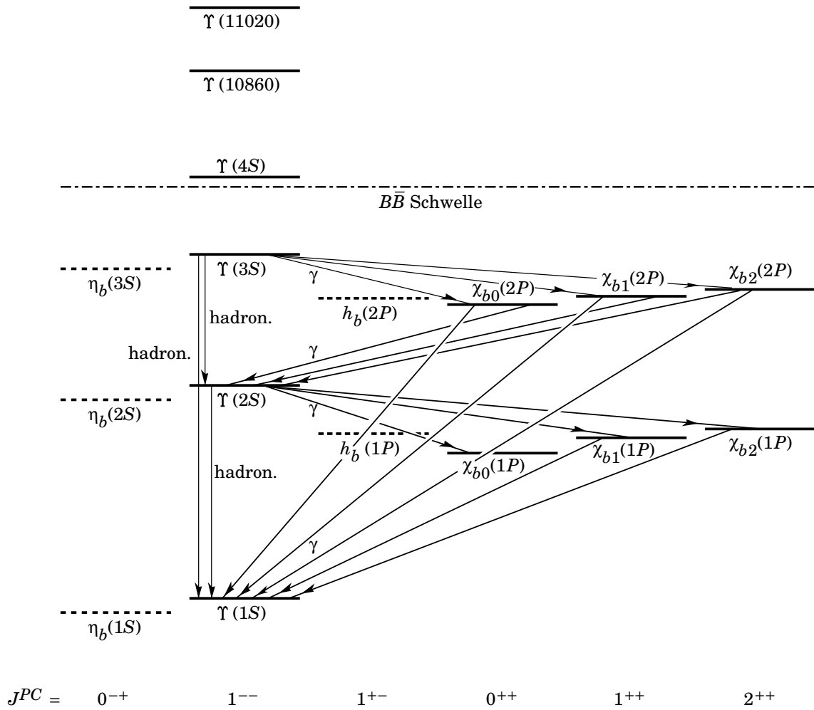
Abbildung 1.2: Termschema des Bottomiums [Gro00]. Die gestrichelten Linien zeigen experimentell noch nicht bestätigte Zustände.
