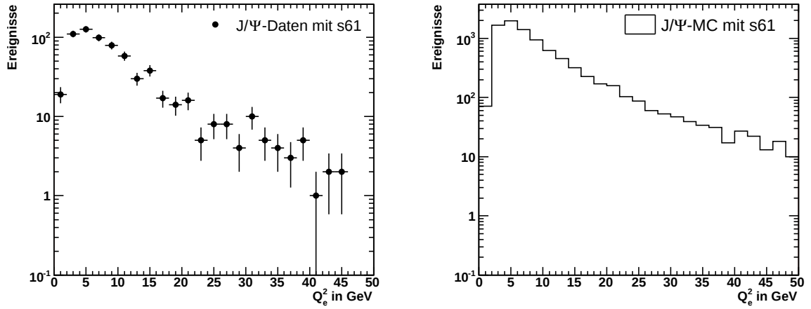
Abbildung 5.19: Verteilung von Q_e^2 der J/\Psi mit s61. Links sind die Daten zu sehen, rechts die MonteCarlo-Simulation für tiefunelastische J/\Psi .
