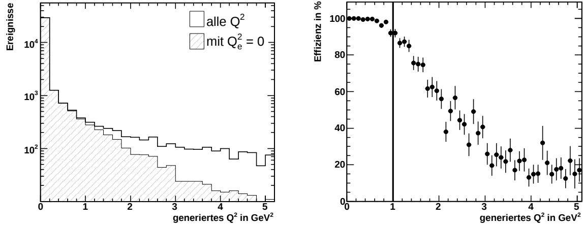
Abbildung 5.13: Verteilung der Q^2 -Werte aus der elastischen Signal-MonteCarlo-Simulation. Schraffiert sind die Ereignisse eingetragen, die die Bedingung Q_e^2 = 0 erfüllen. Rechts ist die Effektivität dieses Schnittes zu sehen.
