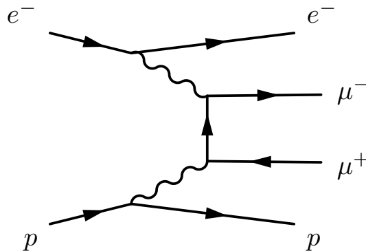
Abbildung 1.5: Dieser reine QED Feynmangraph zeigt den wichtigsten Untergrundprozeß, die Myonpaar-Photoproduktion.
