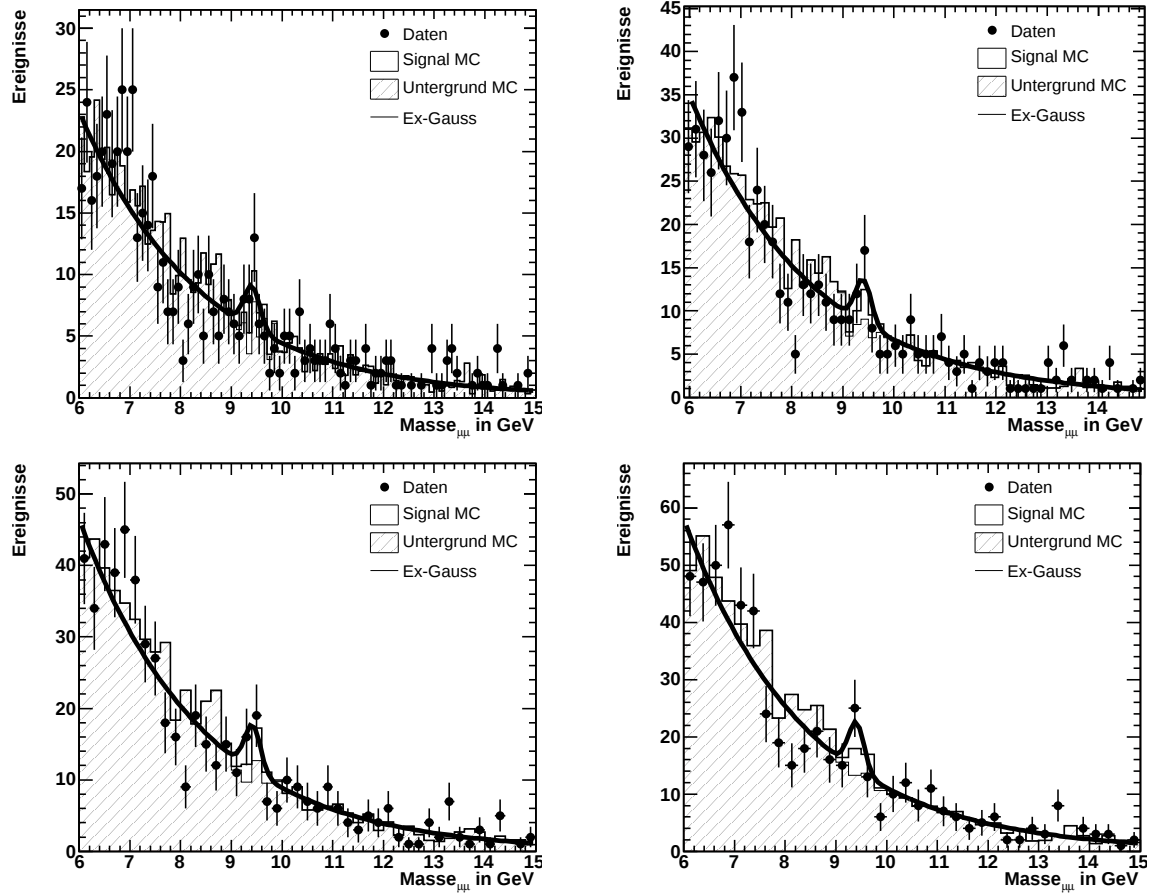
Abbildung 5.4: Anpassung der Daten im Bereich Wgp1 durch die Summe einer Exponential- und einer Gaußfunktion. Die Histogramme zeigen die Anpassungen mit den Binbreiten [100, 150, 200, 250] in MeV. Die Ergebnisse sind in Tabelle 5.3 zu sehen.
