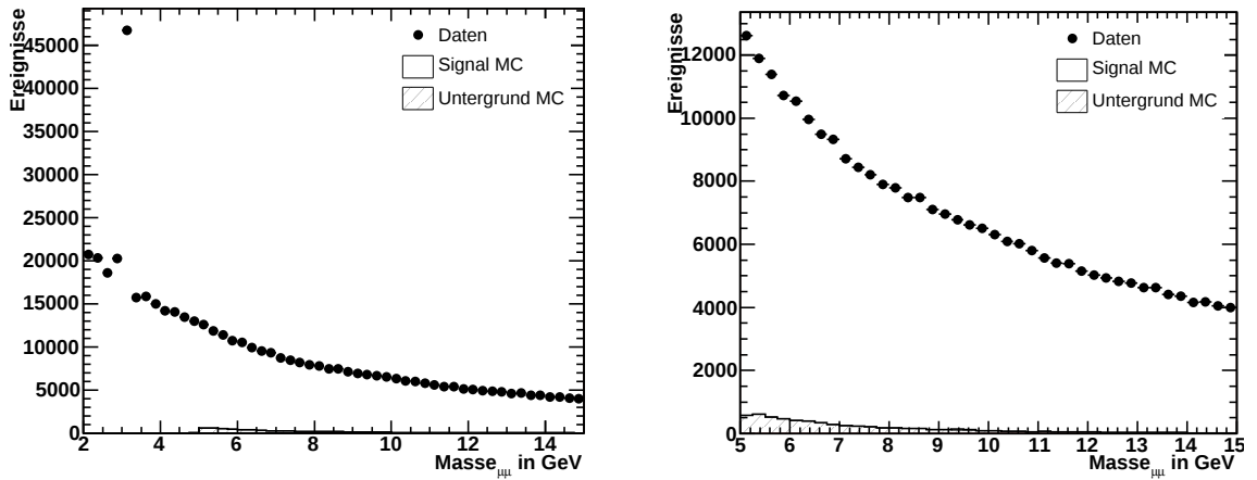
Abbildung 4.3: Massenverteilung nach den Forderungen der Vorselektion
