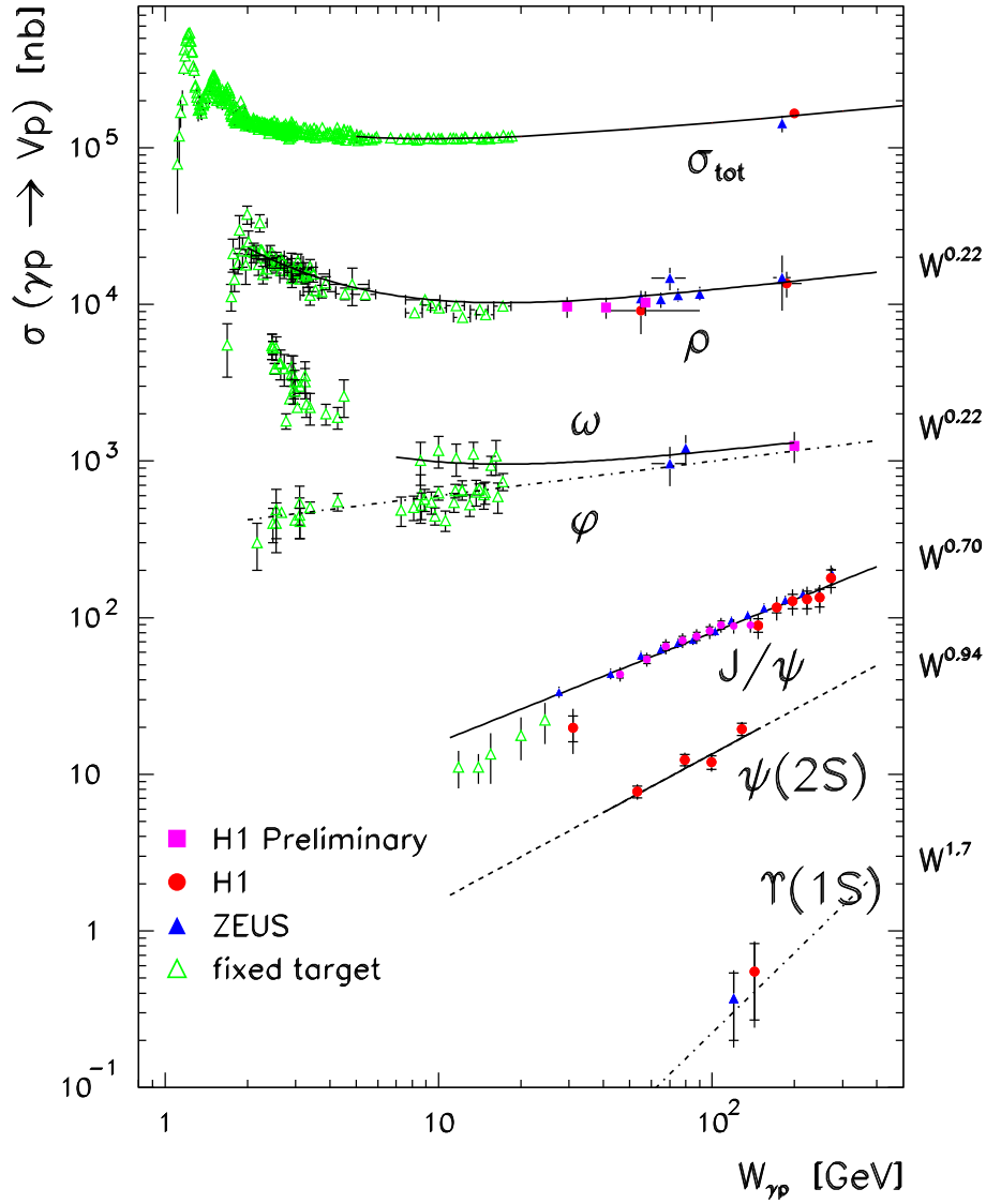
Abbildung 0.1: Wirkungsquerschnitte für diffraktive Vektormesonproduktion und totaler Photoproduktionswirkungsquerschnitt in Photon-Proton-Wechselwirkungen in Abhängigkeit der Photon-Proton-Schwerpunktsenergie W_{\gamma p} .
