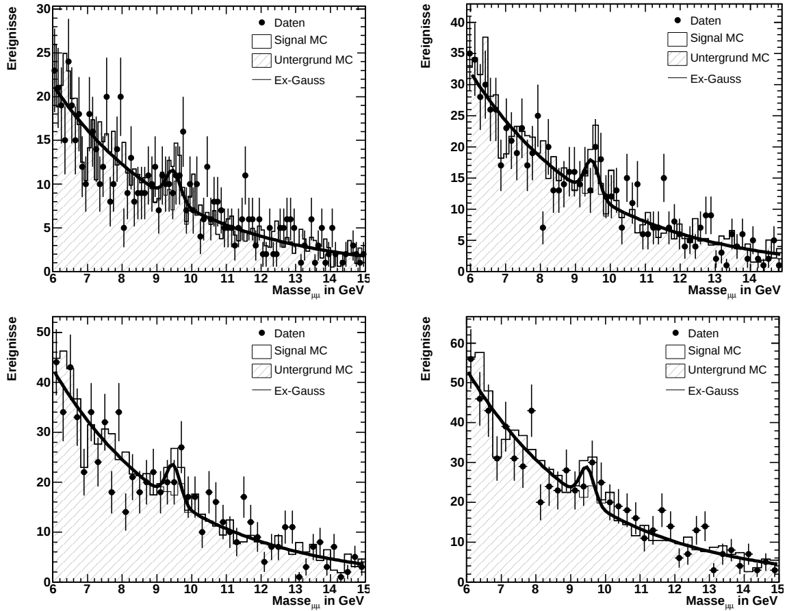
Abbildung 5.7: Anpassung der Daten im Bereich W_{g2} durch die Summe einer Exponential- und einer Gaußfunktion. Dabei wurden die Energieabhängigkeit des Untergrundes, die Resonanzmasse und -breite durch die Werte der MonteCarlo-Simulation fixiert. Die Histogramme zeigen die Anpassungen mit den Binbreiten [100, 150, 200, 250] in MeV. Die Ergebnisse sind in Tabelle 5.4 dargestellt.
