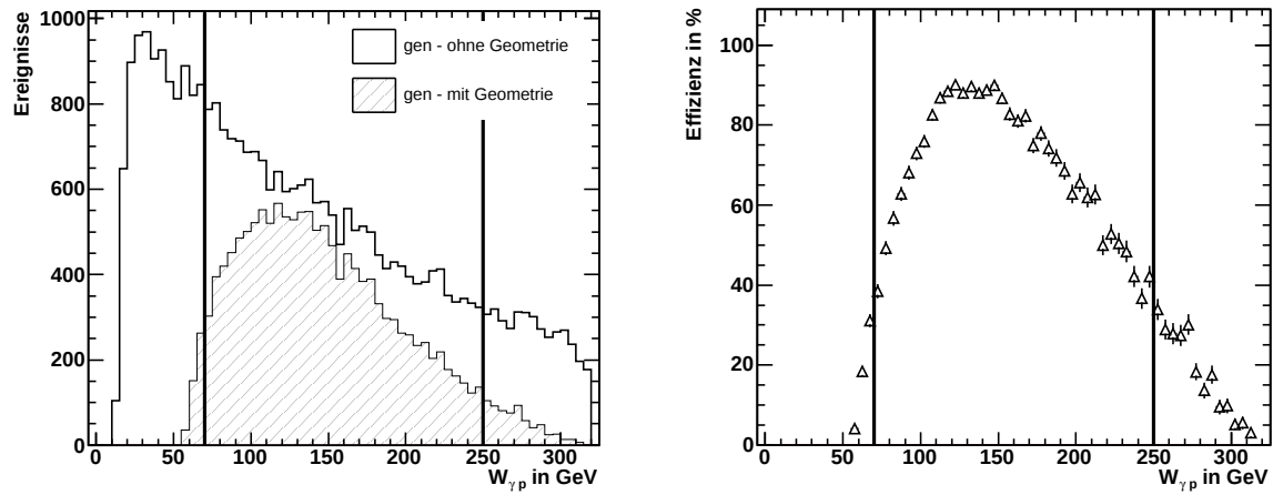
Abbildung 5.14: Geometrische Akzeptanz in Abhängigkeit der Photon-Proton-Schwerpunktsenergie
