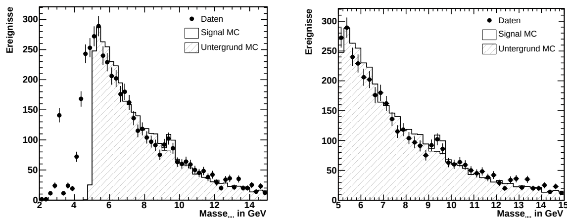
Abbildung 4.11: Massenverteilung nach der Forderung, daß beide Myonen einen Transversalimpuls p_t von mindestens 2.0 GeV besitzen
