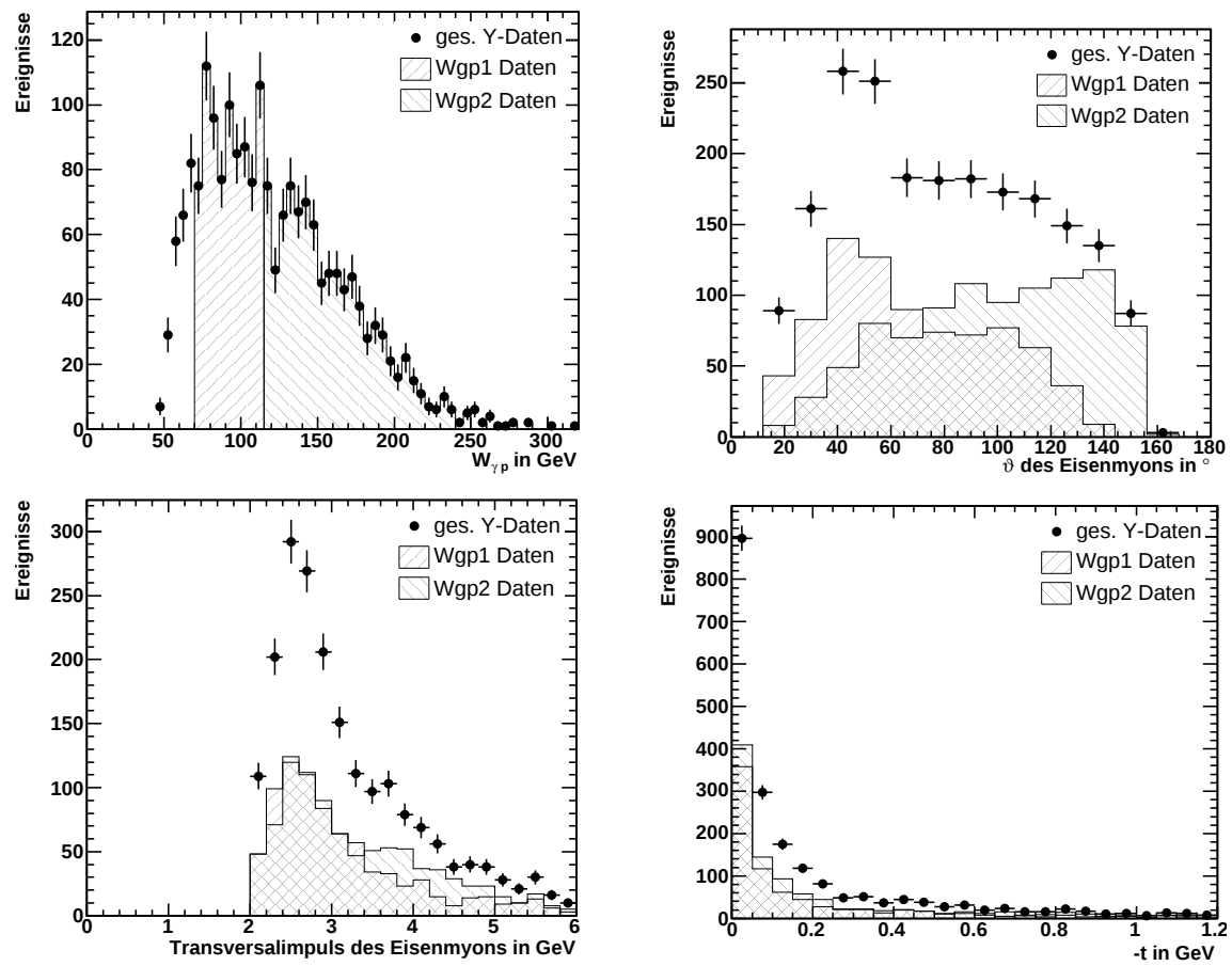
Abbildung 5.23: Verteilungen der charakteristischen Größen der selektierten \Upsilon -Daten
