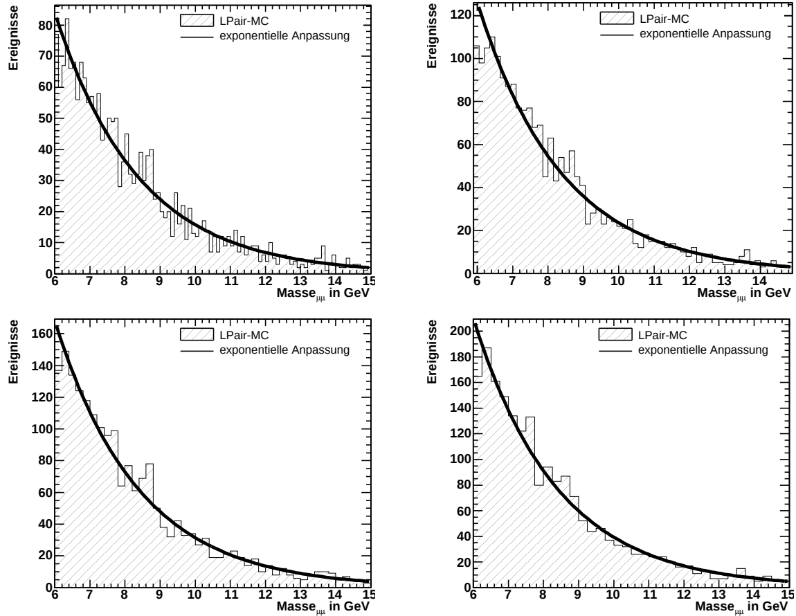
Abbildung 5.2: Anpassung des Untergrundes im Bereich Wgp1, der durch den MonteCarlo-Generator LPair erzeugt wird, mittels einer Exponentialfunktion. Die Histogramme zeigen die Anpassung mit den Binbreiten [100, 150, 200, 250] in MeV. Die Ergebnisse sind in Tabelle 5.2 zu sehen.
