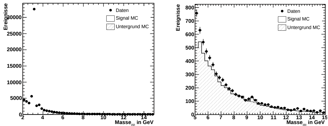
Abbildung 4.7: Massenverteilung nach den ersten Schnitten gegen den nicht ep -induzierten Untergrund
