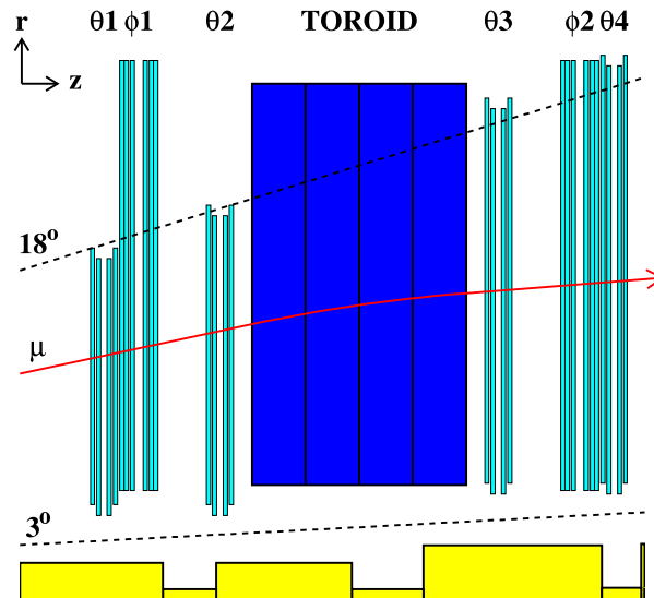
Abbildung 2.7: Das Vorwärts-Myonsystem im Querschnitt
