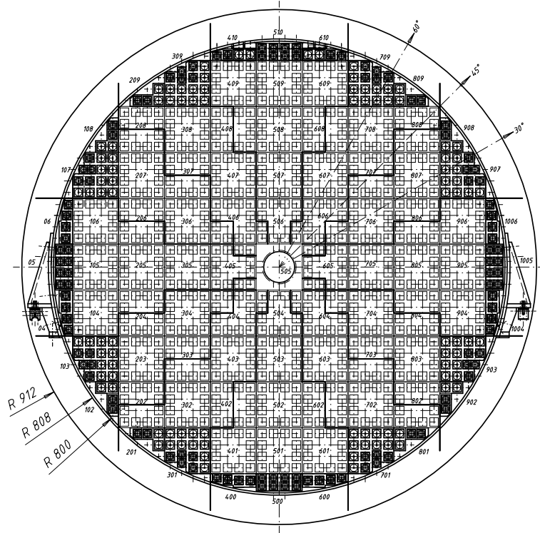
Abbildung 2.5: Ansicht des Spaghetti-Kalorimeters in der r\varphi -Ebene
