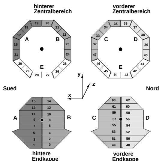
Abbildung 4.1: Einteilung des Myonsystems in Sektoren. Zum inneren Teil der Endkappe gehören die Segmente 6-11 bzw. 54-59. Die Segmente 0-5 und 12-15 bzw. 48-53 und 60-63 bilden den äußeren Teil des Myonendkappensystems.
