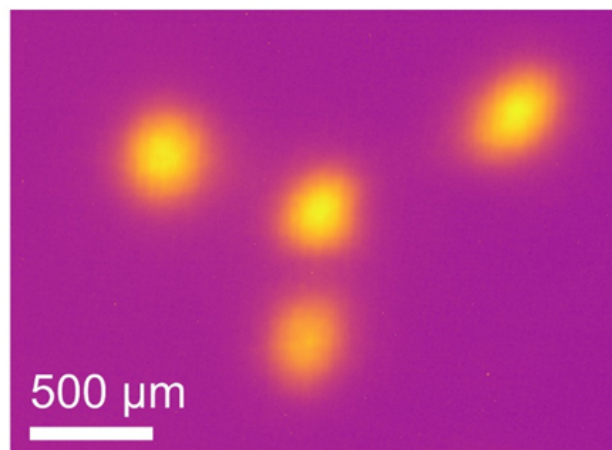
Abbildung 5.2: Abbild der BESSY II-Strahlungsquellpunkte im Zwei-Orbit-Modus. Der zweite Orbit windet sich um den Standardorbit im Zentrum und schließt sich nach drei Umläufen (entsprechend den 3 äußeren Punkten). Die verschiedenen Orbits erlauben es, unterschiedliche Nutzerexperimente mit dem jeweils passenden Licht gleichzeitig zu versorgen.
