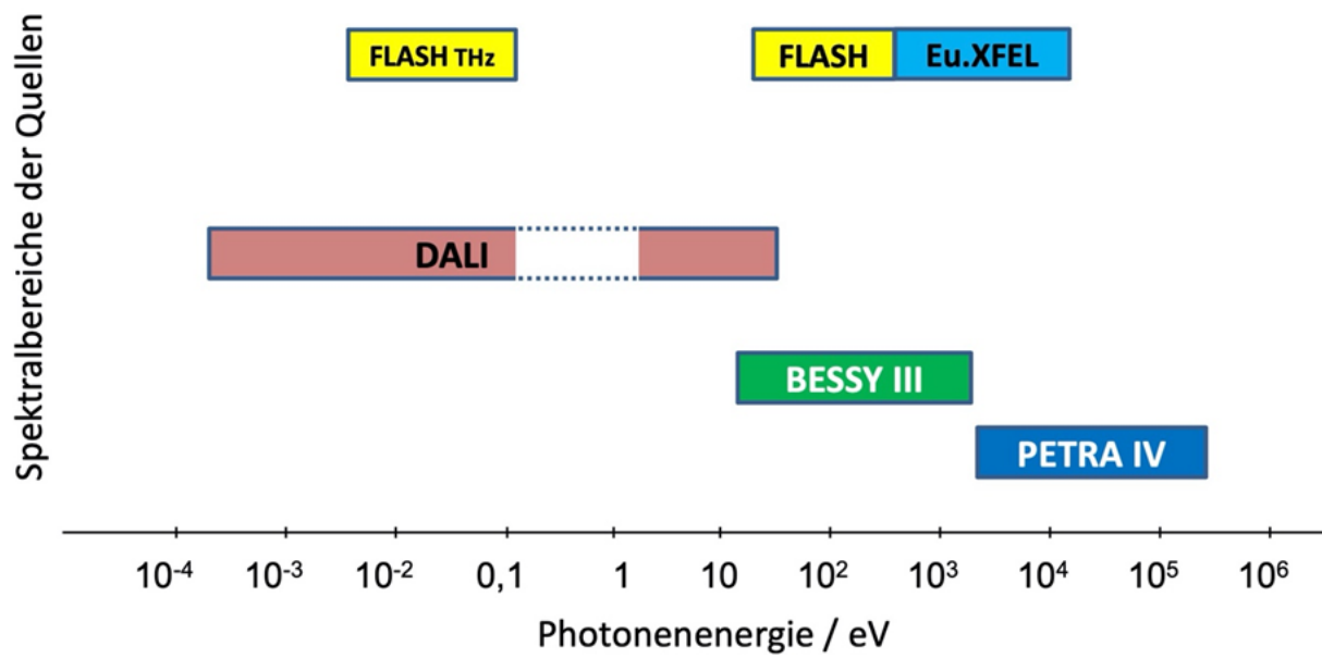
Abbildung 5.1: Schematische Darstellung der Kernphotonenenergiebereiche der von der Helmholtz-Gemeinschaft betriebenen und geplanten Synchrotron- und FEL-Strahlungsquellen, einschließlich des European XFEL. Die komplementären Photonenenergiebereiche der Quellen BESSY II/III und PETRA III/IV werden durch die Upgrades beibehalten. Die komplementären Betriebsarten DALI (CW-Betrieb) und FLASH (Pulsfolgenbetrieb) für VUV/Soft-X Pump & Probe-Sonden-Experimente erhöhen die Vielfalt der möglichen Anwendungen erheblich. Die erreichbare Zeitauflösung an Speicherring-quellen reicht bis in den sub-Nanosekundenbereich. Mit den FELs (FLASH und European XFEL) ist man in der Lage, bis in den sub-10-Femtosekundenbereich vorzustoßen.
