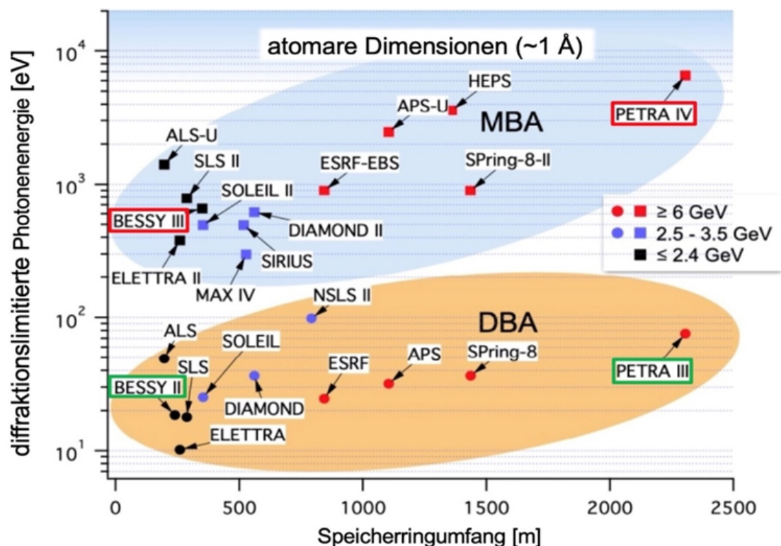
Abbildung 6.1: Darstellung der Photonenenergie, bis zu der eine Quelle beugungsbegrenzt ist, d.h. bis zu der Photonenenergie die theoretisch mögliche Brillanz erreicht wird, als Funktion des Umfangs. DBA: Double-Bend-Achromat, Quellen der 3. Generation; MBA: Multi-Bend-Achromat, Quellen der 4. Generation. DALI ist hier, da kein Speicherring, nicht aufgeführt (ein internationaler Vergleich ist in Tabelle 6.3 zu finden).
