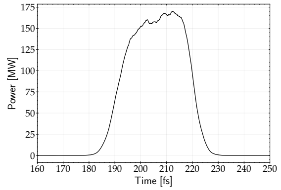
(d) Power Profile after 5 modules of the amplifier.
