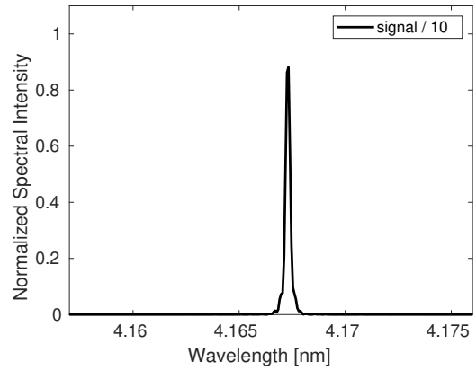
(d) Oscillator-FEL starting from shot-noise.
