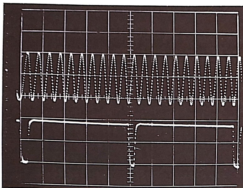
Bild 23 Ein- und Ausgangsspannung einer schnellen Untersetz- dekade
