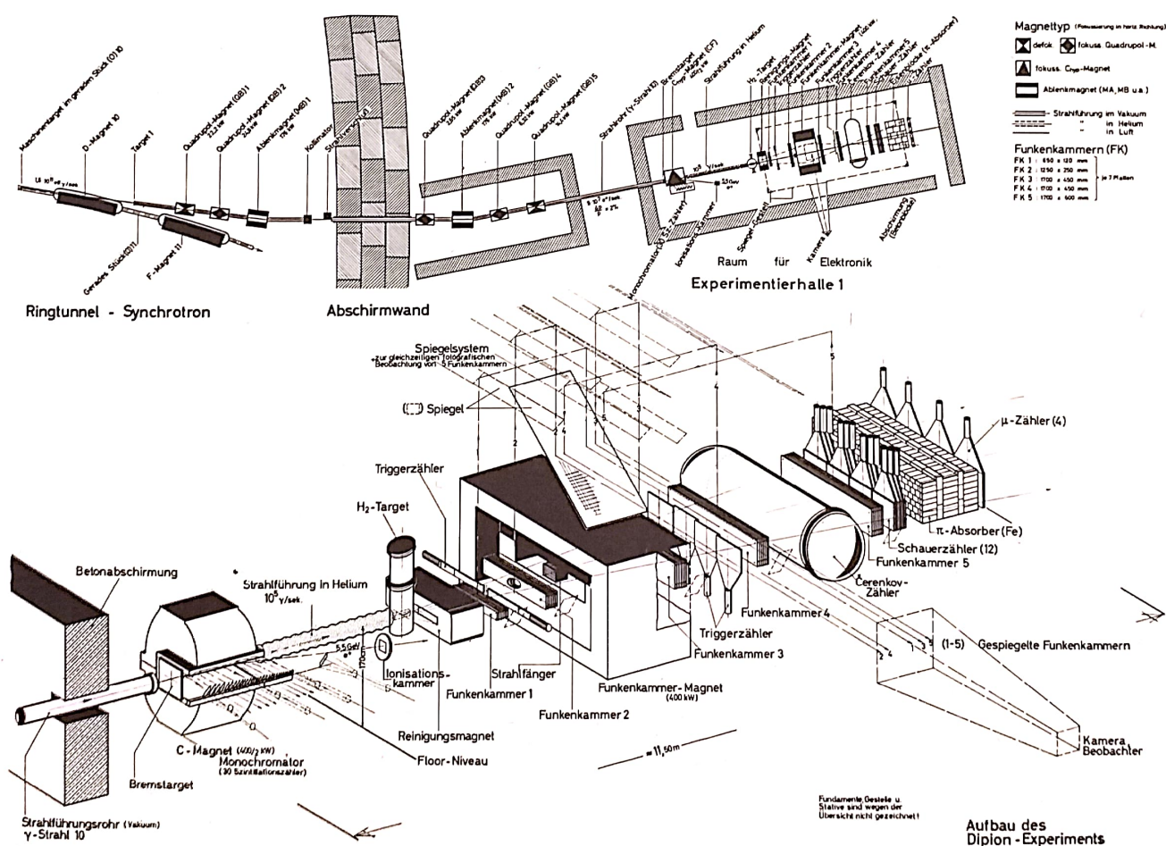
Bild 11 Strahlaufbau und Schema der Experimentier-Anordnung F 32
