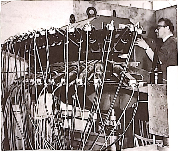
Bild 12 Monochromator
