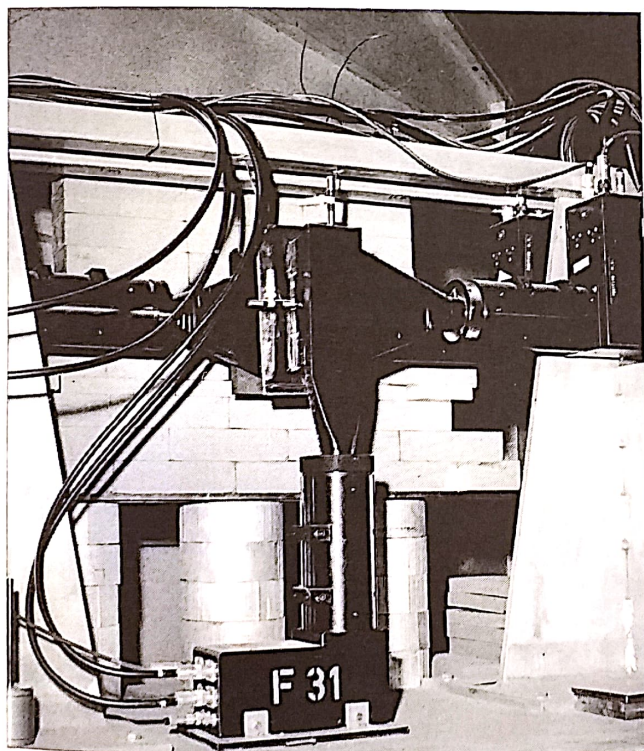
Bild 9 Protonen-Reichweiten-Teleskop
