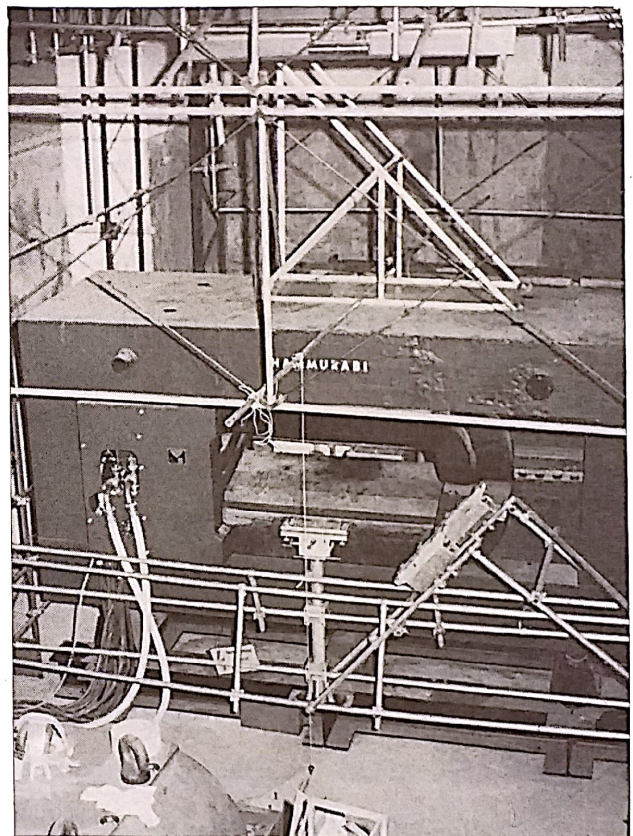
Bild 22 Der 80 Tonnen schwere Ablenkmagnet für das Funkenkammer-Experi- ment
