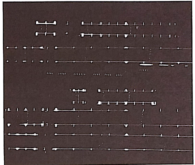
Bild 13 Funkenkammer-Aufnahme mit einem Elektroproduktions-Ereignis
