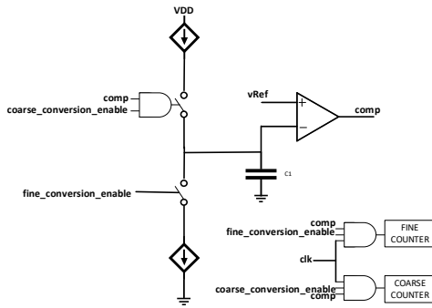
Fig. 5. ADC schematic
