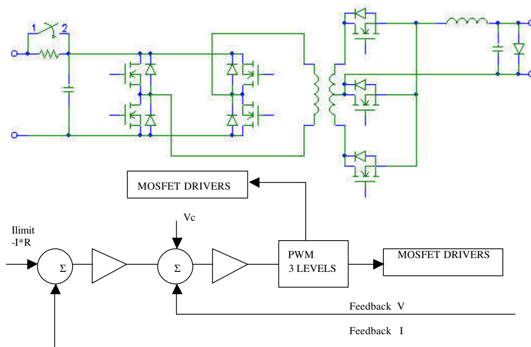
Figure 5.1.- d.c/d.c. Module 25 A ( Input 400 Vdc. Output 0 to +10 V dc)
