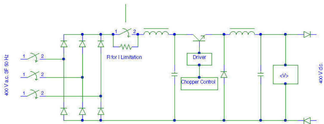
Figure 5.5. Input Module a.c./d.c.
