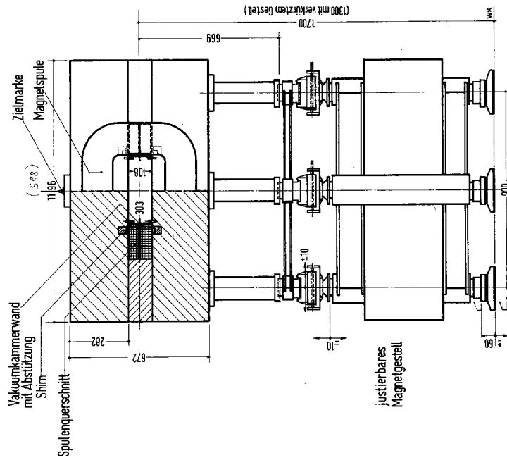
Querschnitt Ablenk magnet Typ: MB
