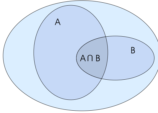
Fig. 2.1. Venn diagram.
