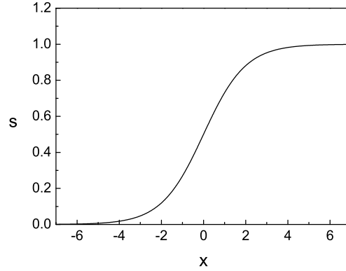
Fig. 11.10. Sigmoid funktion.
