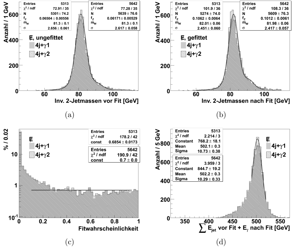
Abbildung 5.10: p_x, p_y fest kontra p_x, p_y frei auf der Teilmenge „E“: Vergleich analog zu Abb. 5.9. Erfolgsquote: 36%/38%; \Delta m_W : +0.7 GeV/+0.7 GeV; \Delta\sigma : -0.2 GeV/-0.2 GeV für 4j+γ1/4j+γ2.
