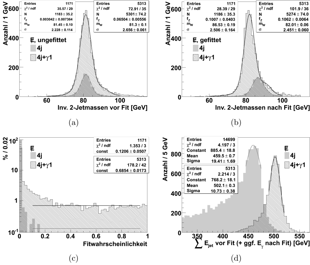
Abbildung 5.3: Fits mit und ohne Photon auf der Teilmenge „E“: Hier wird der bereits bekannte 4-Jet-Fit ((5C,) 4j; grau) mit einem Fit verglichen, der zusätzlich ein Photon mit einer freien Impulskomponente p_z enthält (4j+γ1; schraffiert). Beide Fits enthalten die fünf Nebenbedingungen gemäß Tab. 3.1. (a) zeigt den Mittelwert der invarianten 2-Jet-Massen vor dem Fit, (b) eben diesen nach dem Fit, (c) die Fitwahrscheinlichkeit, (d) die Summe der ungefiteten Jetenergien plus ggf. der gefitteten Photonenergie. Erfolgsquote: 8%/36%; \Delta m_W : +5 GeV/+0.7 GeV; \Delta \sigma : +0.3 GeV/−0.2 GeV für 4j/4j+γ1.
