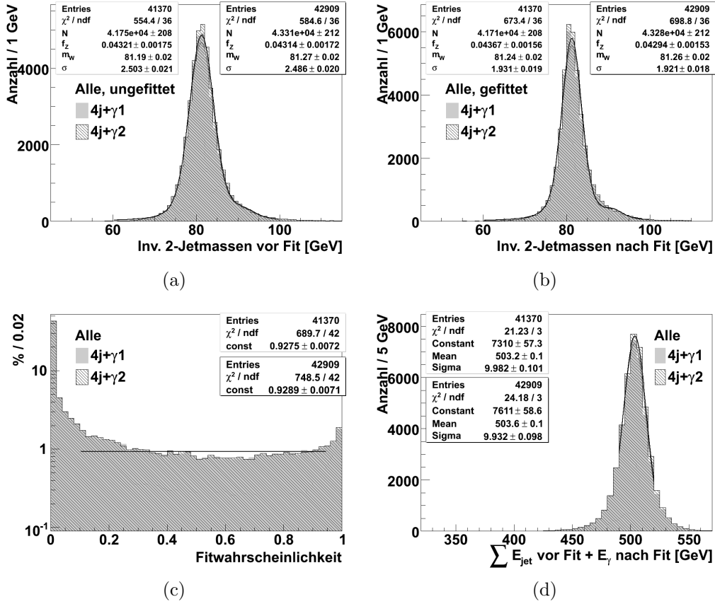
Abbildung 5.9: p_x, p_y fest kontra p_x, p_y frei auf dem vollständigen Datensatz: Hier wird der 4-Jet-Fit mit fünf Nebenbedingungen für zwei verschiedene Photonfitobjekte verglichen. 4j+γ1 (grau) hat nur den freien Parameter p_z , während bei 4j+γ2 (schraffiert) alle drei Impulskomponenten variiert werden können ( \sigma_{p_x} = \sigma_{p_y} = 0.2 GeV). (a) zeigt den Mittelwert der invarianten 2-Jet-Massen vor dem Fit, (b) ebendiesen nach dem Fit, (c) die Fitwahrscheinlichkeit, (d) die Summe der ungefiteten Jetenergien plus ggf. der gefitteten Photonenergie. Erfolgsquote: 61 %/63 %; \Delta m_W : +0.1 GeV/±0.0 GeV; \Delta \sigma : -0.6 GeV/-0.6 GeV für 4j+γ1/4j+γ2.
