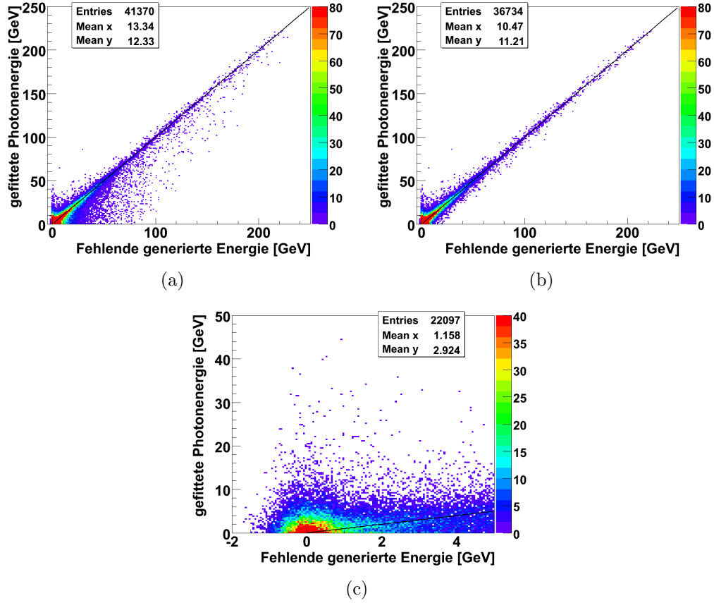
Abbildung 5.2: Vergleich der gefitteten Photonenergie mit der fehlenden Energie auf Generator-Ebene für ein Photon mit freiem p_z . (a) zeigt die vollständige Verteilung, (b) mit dem zusätzlichen Schnitt \sum E_{\text{fehl}}^{\text{gen}} - |\sum p_z^{\text{fehl,gen}}| < 5 GeV. (c) zeigt den Ausschnitt aus (a) für E_{\text{fehl}}^{\text{gen}} < 5 GeV.
