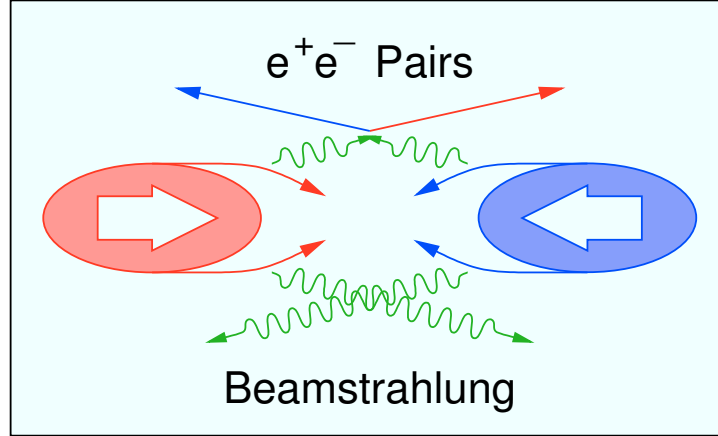
Abbildung 2.5: Schematische Darstellung des Pinch-Effekts: Zwei Elektronenpakete kurz vor der Kollision. Die äußeren Elektronen werden durch das Feld des entgegenkommenden Paketes nach innen abgelenkt und strahlen dabei Photonen ab. Diese Abbildung wurde freundlicherweise von Adrian Vogel zur Verfügung gestellt.
