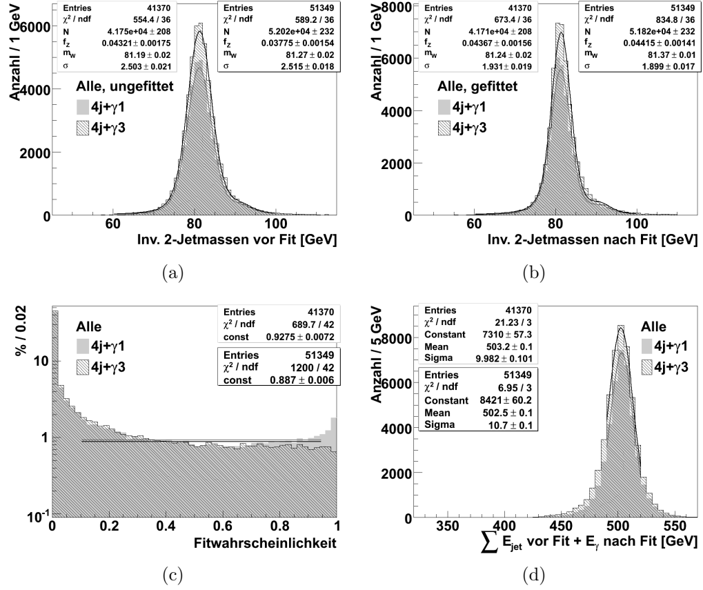
Abbildung 5.15: Gauß-Verteilung kontra Näherung durch Potenzfunktion auf dem vollständigen Datensatz: Hier wird der 4-Jet-Fit mit fünf Nebenbedingungen für zwei verschiedene Photonfitobjekte mit freiem Parameter p_z verglichen. 4j+γ1 (grau) ist die bekannte Version mit dem durch eine Gauß-Verteilung beschriebenen Impulsspektrum, während bei 4j+γ3 (schraffiert) das Spektrum durch eine Potenzfunktion (Abb. 5.12) beschrieben wird. (a) zeigt den Mittelwert der invarianten 2-Jet-Massen vor dem Fit, (b) ebendiesen nach dem Fit, (c) die Fitwahrscheinlichkeit, (d) die Summe der ungefiteten Jetenergien plus der gefitteten Photonenergie. Erfolgsquote: 61 %/75 %; \Delta m_W : +0.1 GeV/+0.1 GeV; \Delta \sigma : -0.6 GeV/-0.6 GeV für 4j+γ1/4j+γ3.
