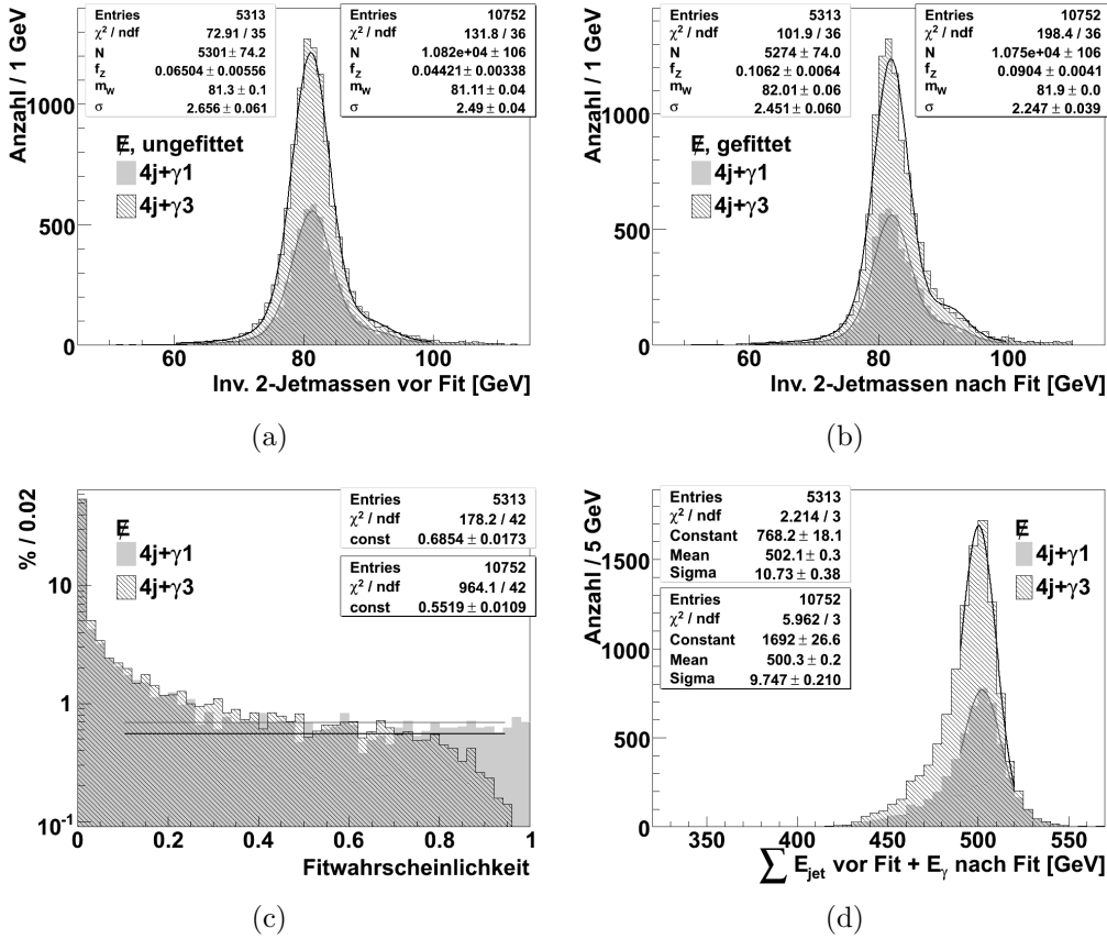
Abbildung 5.16: Gauß-Verteilung kontra Näherung durch Potenzfunktion auf der Teilmenge „ \bar{E} “: Vergleich analog zu Abb. 5.15. Erfolgsquote: 36%/73%; \Delta m_W : +0.7 GeV/+0.8 GeV; \Delta \sigma : -0.2 GeV/-0.2 GeV für 4j+\gamma 1/4j+\gamma 3 .
