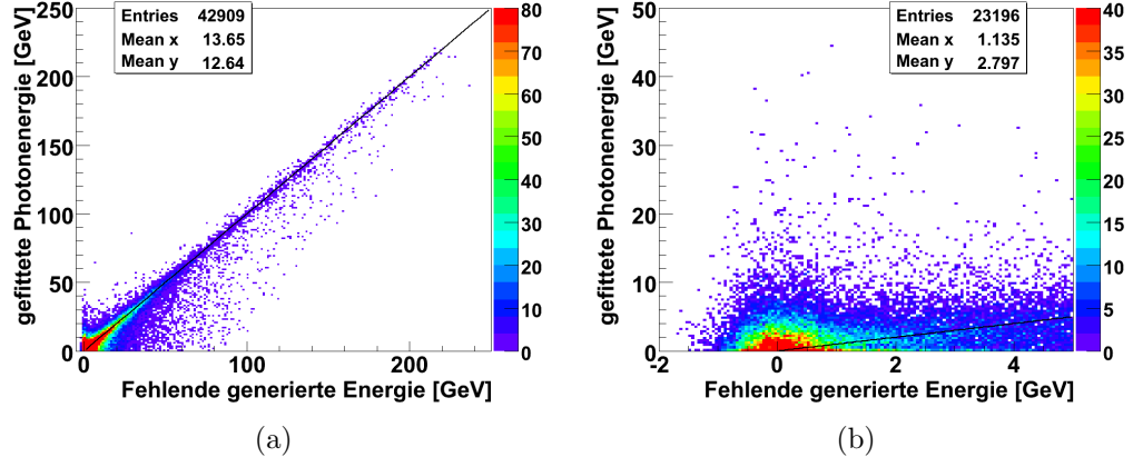
Abbildung 5.8: Vergleich der gefitteten Photonenergie mit der fehlenden Energie auf Generator-Ebene für ein Photon mit freiem p_x, p_y, p_z ( \sigma_{p_x} = \sigma_{p_y} = 0.2 GeV). (a) zeigt die vollständige Verteilung, (b) den Ausschnitt aus (a) für E_{\text{fehl}}^{\text{gen}} < 5 GeV.
