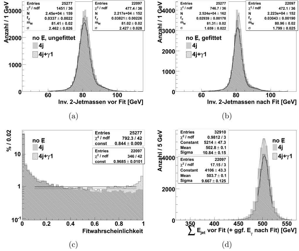
Abbildung 5.4: Fits mit und ohne Photon auf der Teilmenge „no E “: Vergleich analog zu Abb. 5.3. Erfolgsquote: 77%/67%; \Delta m_W : -0.1 GeV/ -0.1 GeV; \Delta\sigma : -0.8 GeV/ -0.6 GeV für 4j/4j+\gamma 1 .
