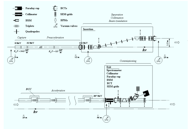
Fig.1 The general PPA scheme.
