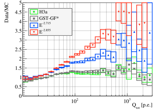
(d) Q_{\text{tot}} , High-Quality Tracks
