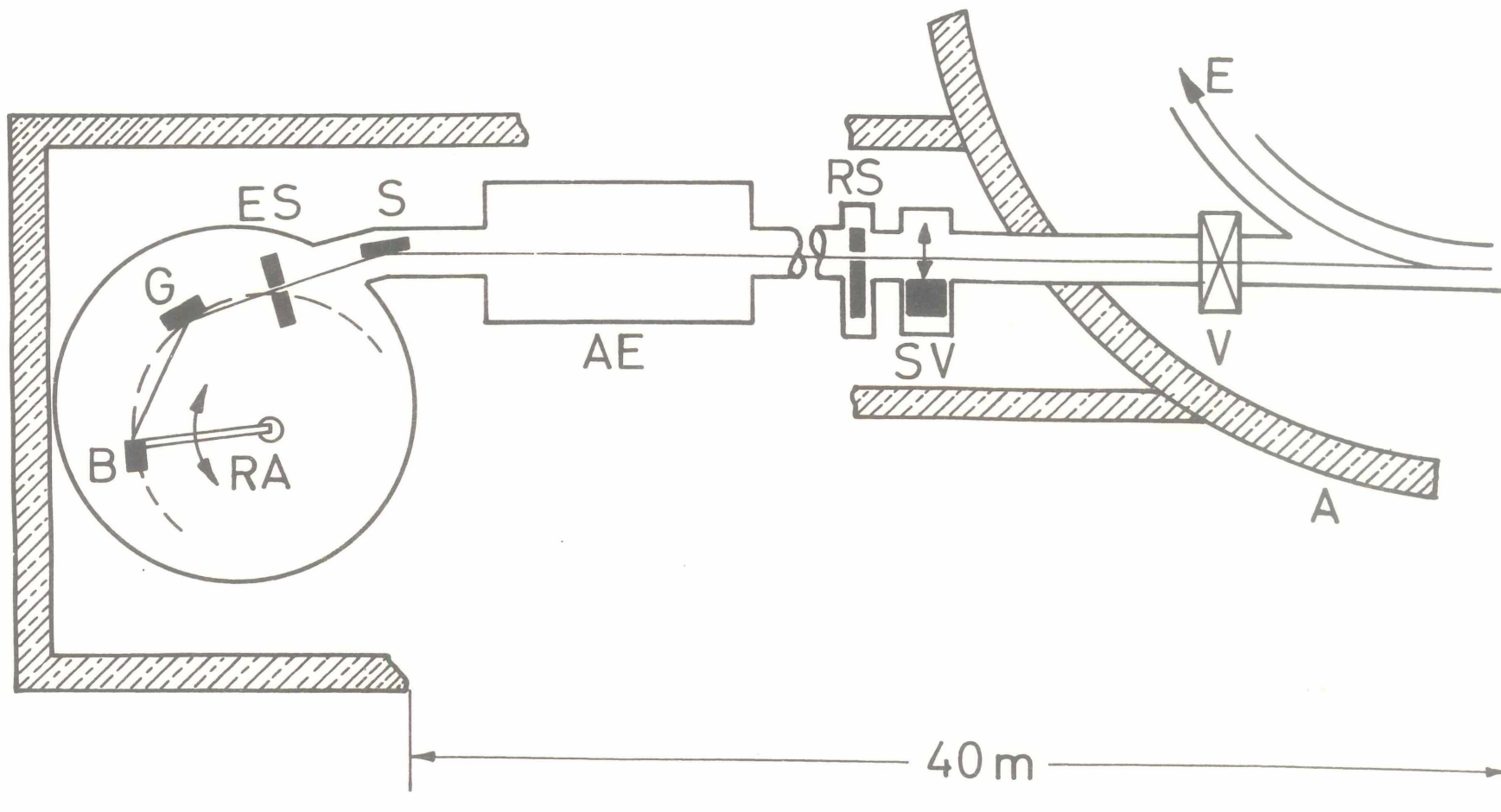
Abbildung 4 : Strahlengang des Synchrotronlichtes (V Ventil, A Abschirmwand, SV Strahlverschuß, RS Rotierende Scheibe, AE Aufdampfgerät, S Spiegel, ES Eintrittsspalt, G Gitter, B Bendix-Photomultiplier, RA schwenkbarer Rowlandarm
