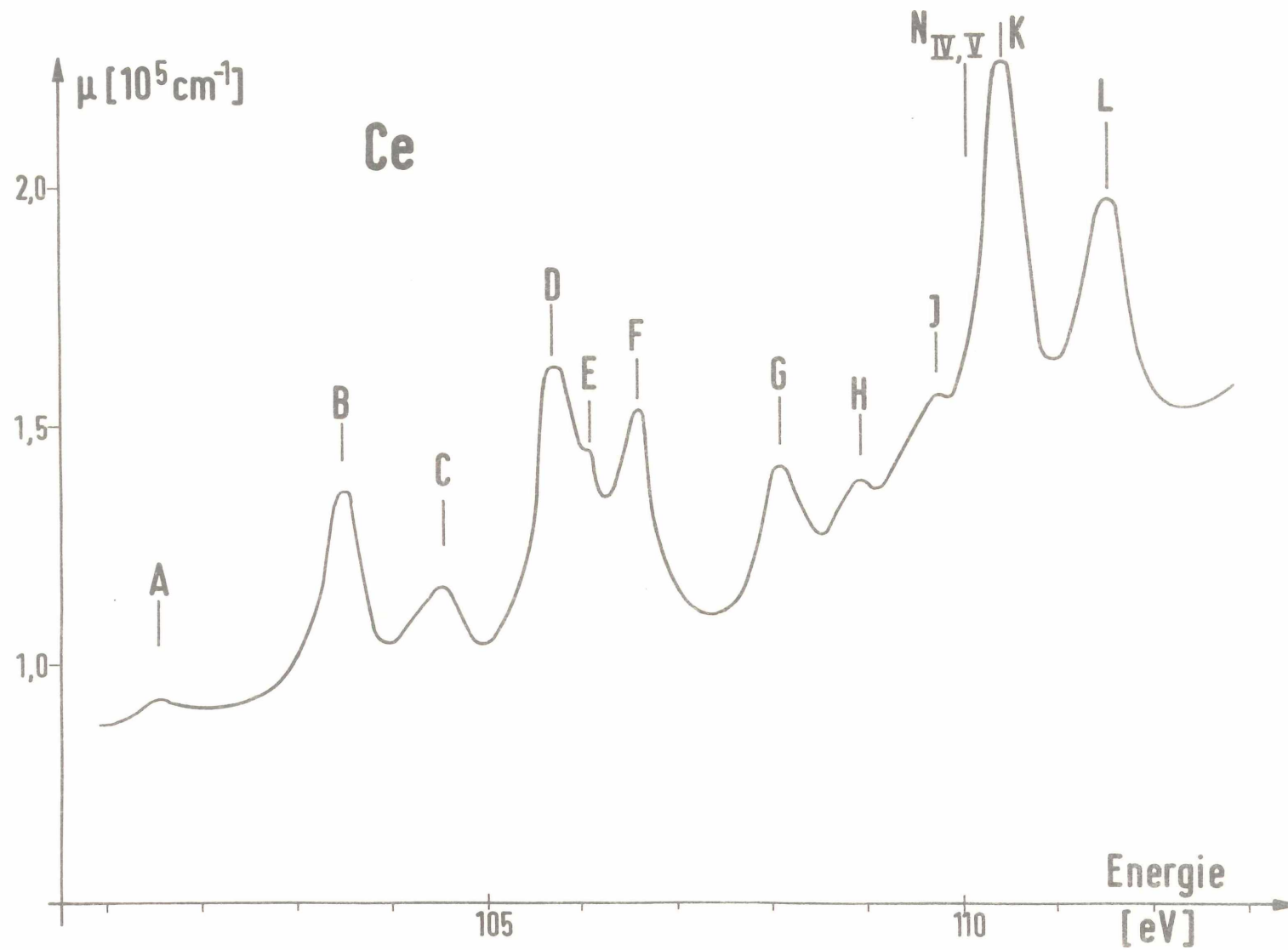
Abbildung 10 : Feinstruktur im Cerspektrum
