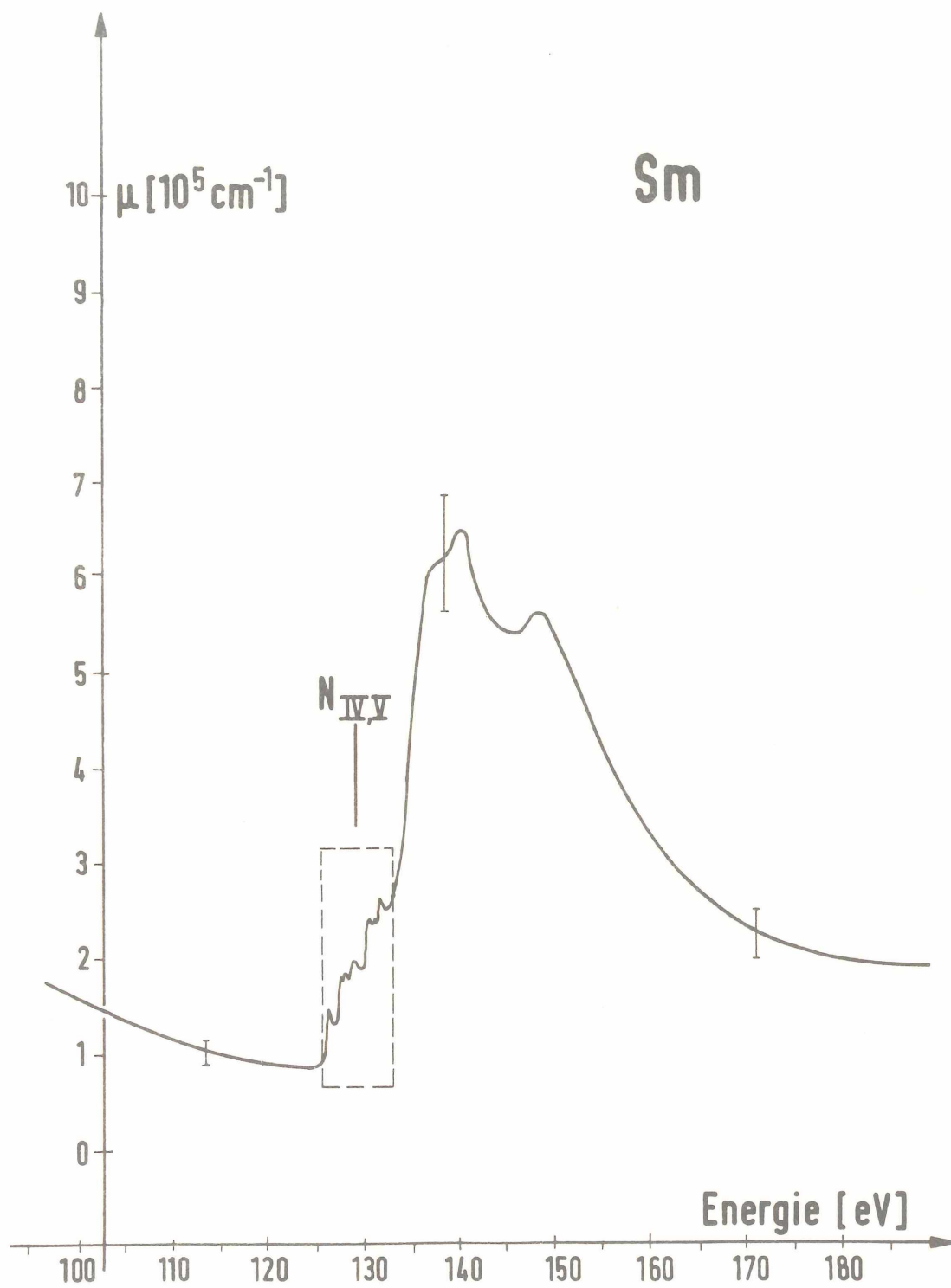
Abbildung 17 : Absorptionsspektrum von Samarium
