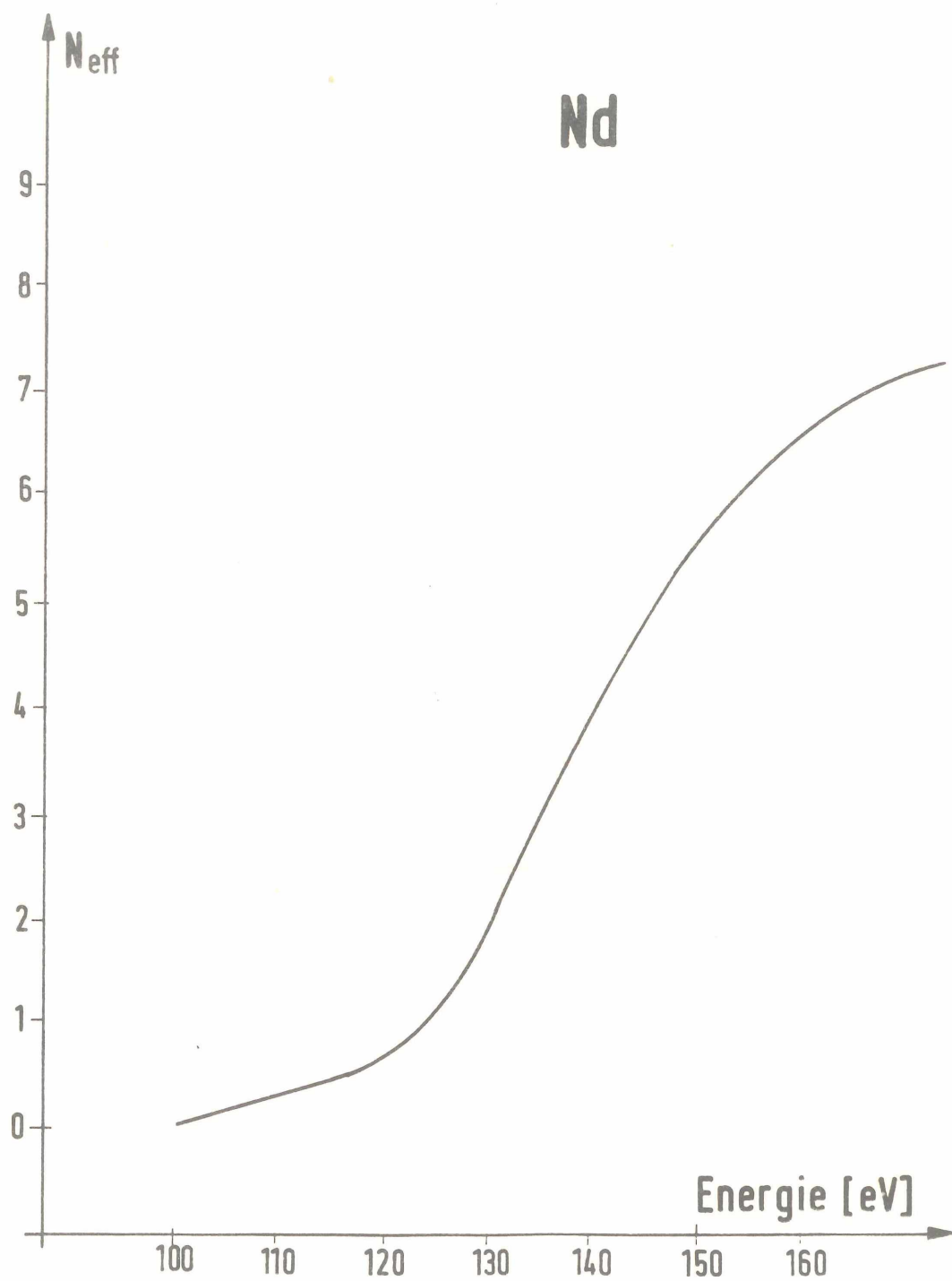
Abbildung 15a : Zahl der effektiven Elektronen (Neodym)
