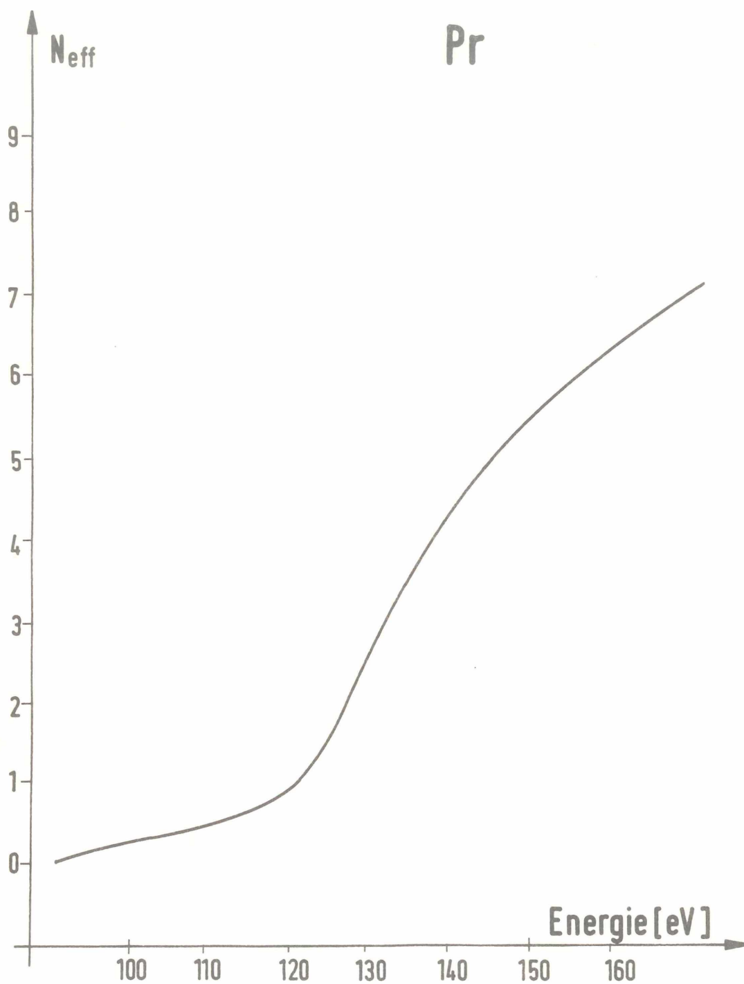
Abbildung 13a : Zahl der effektiven Elektronen (Praseodym)
