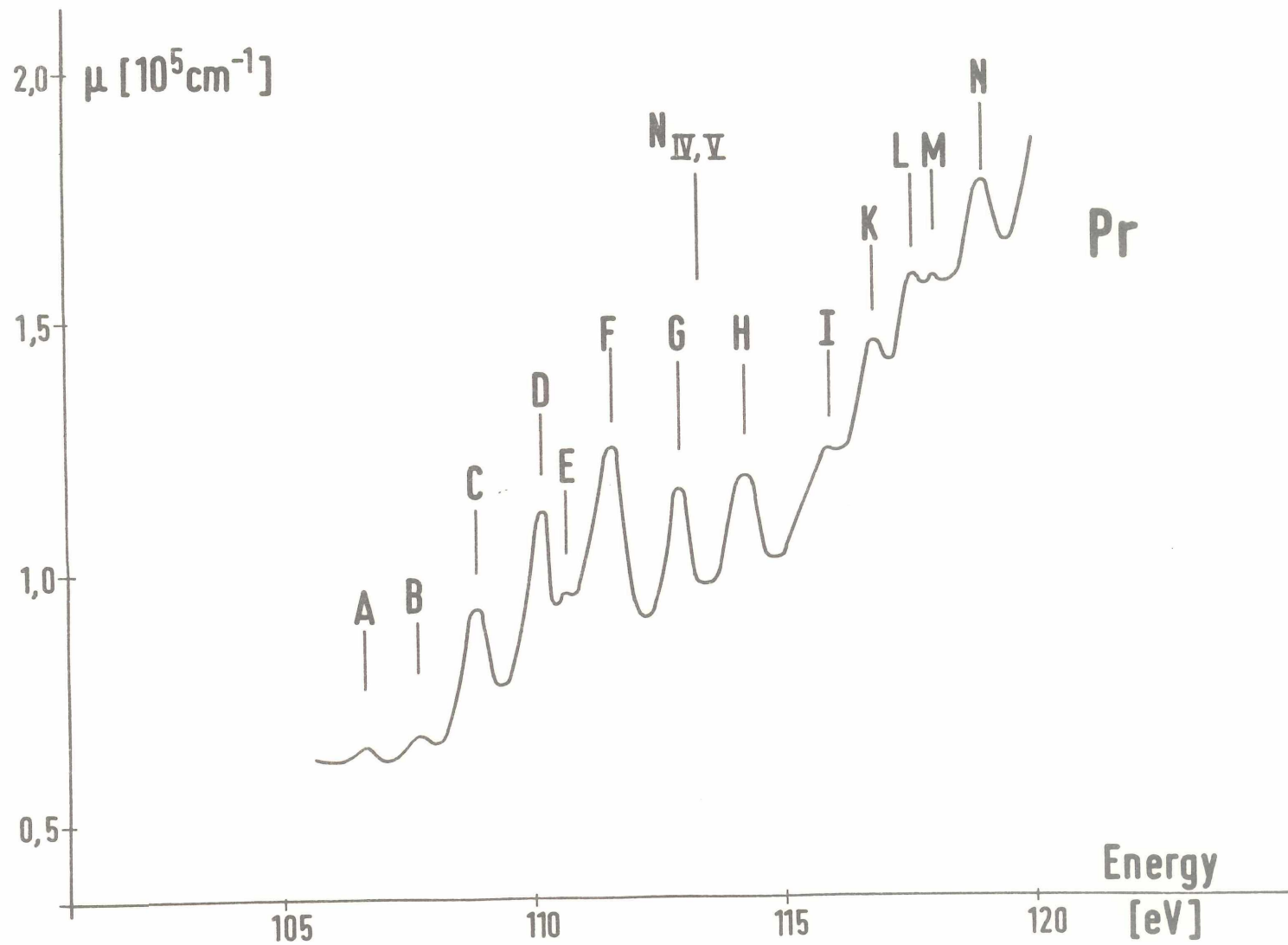
Abbildung 14 : Feinstruktur im Praseodymspektrum
