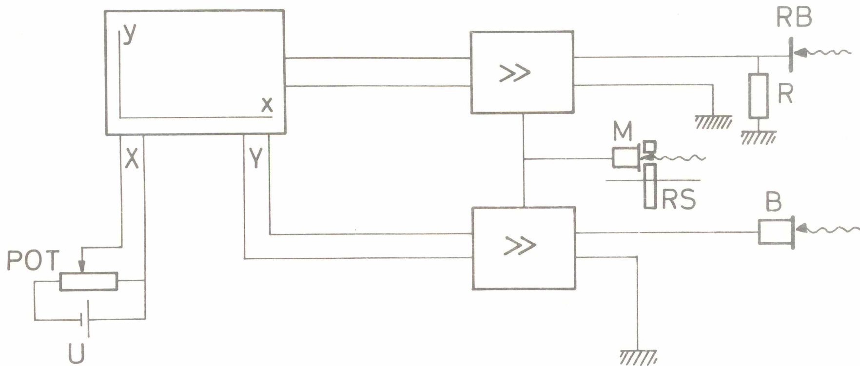
Abbildung 5 :Elektronische Schaltung ( RB Referenzblech,R Widerstand,RS Rotierende Scheibe, M Multiplier,B Bendix-Photomultiplier,POT Potentiometer )
