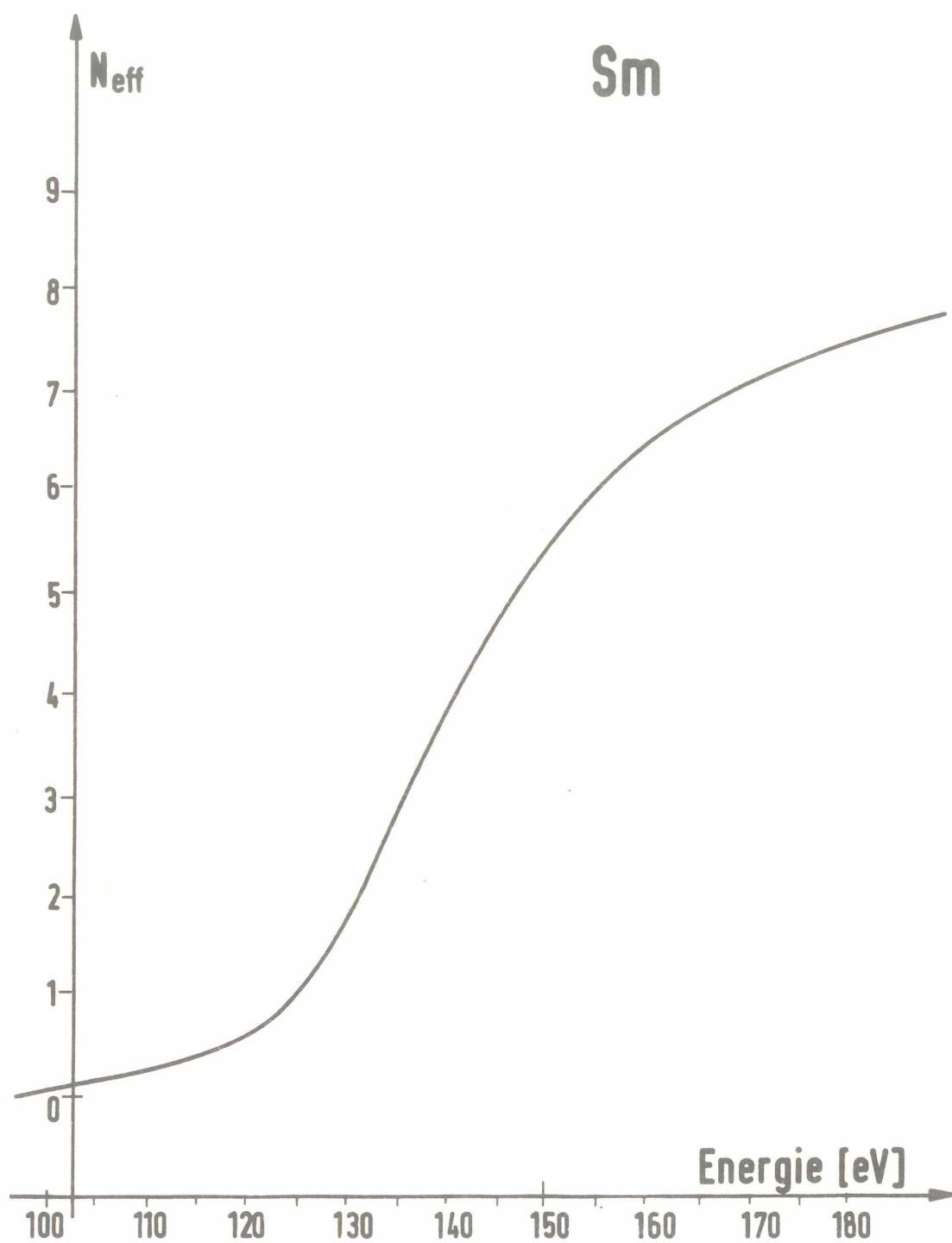
Abbildung 17a : Zahl der effektiven Elektronen (Samarium)
