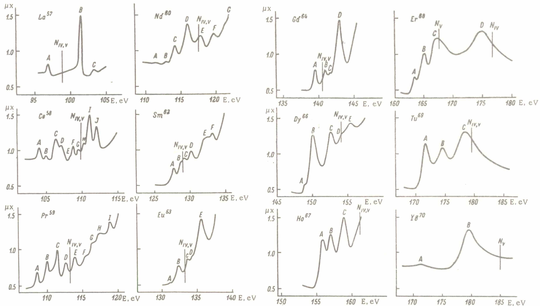
Abbildung 20 : Feinstruktur in den Absorptionsspektren der Lanthaniden
