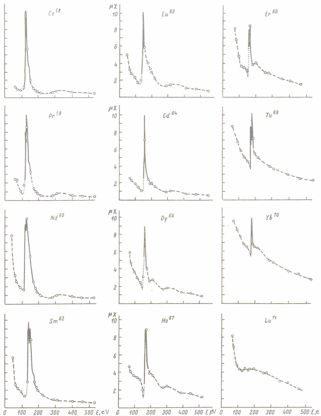
Abbildung 19 : Absorptionsspektren der Lanthaniden
