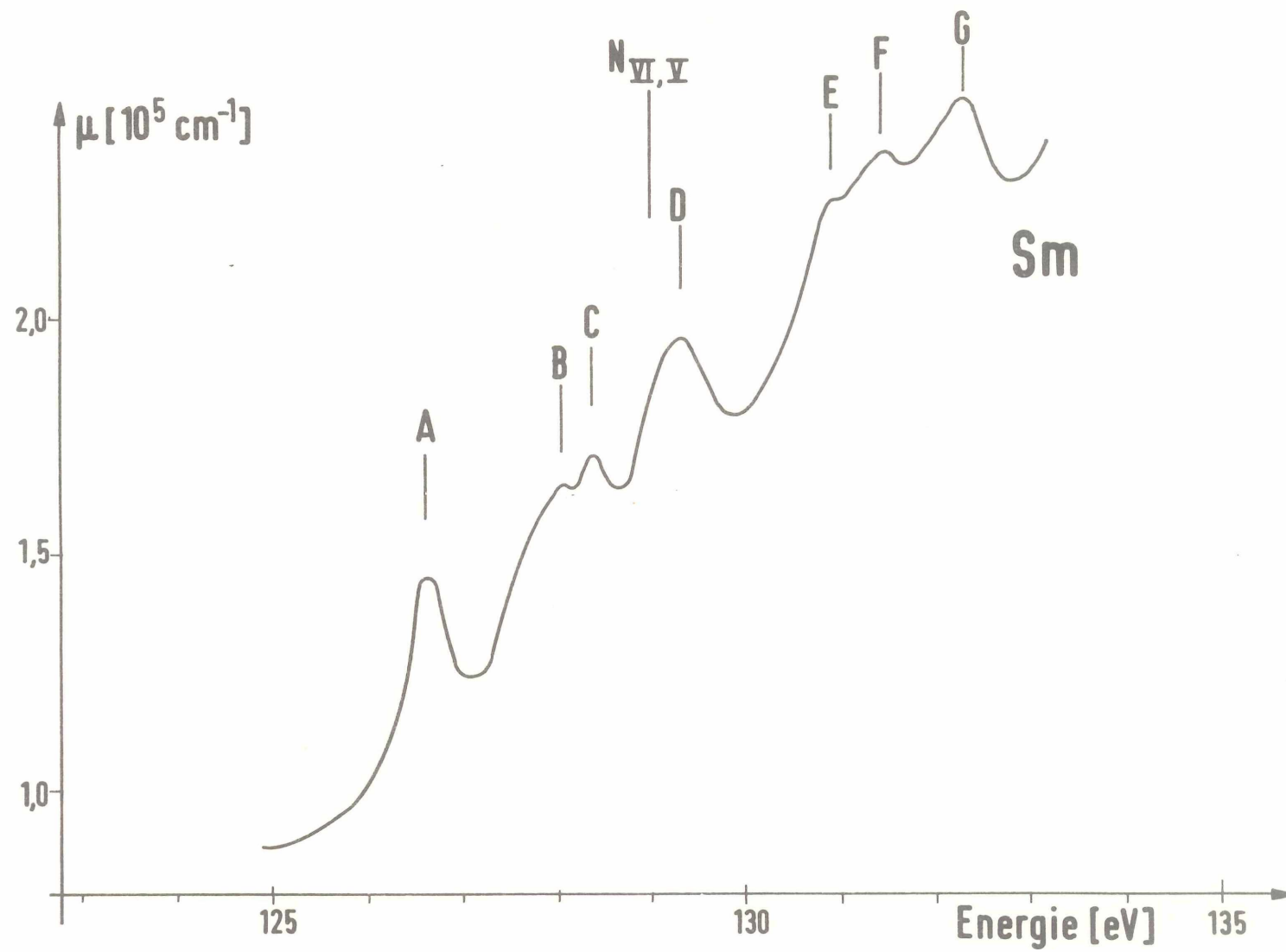
Abbildung 18 : Feinstruktur im Samariumspektrum
