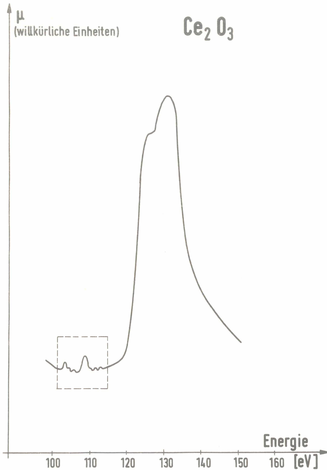
Abbildung 11 : Absorptionsspektrum von Ceroxyd
