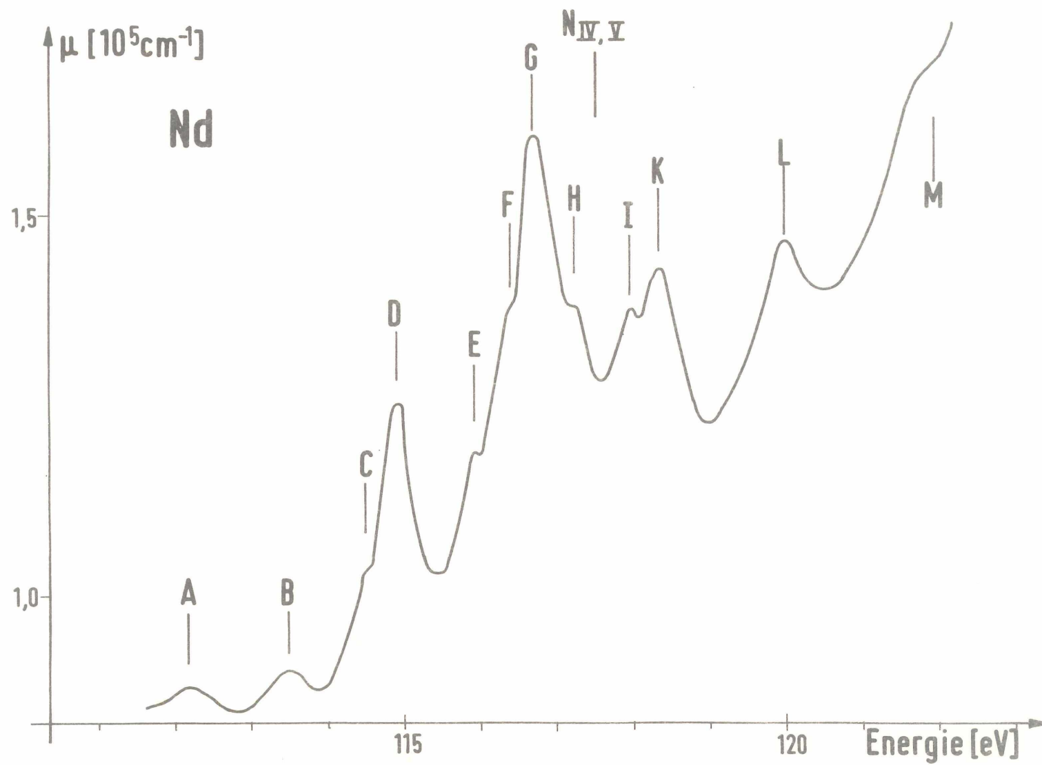
Abbildung 16 : Feinstruktur im Neodymspektrum
