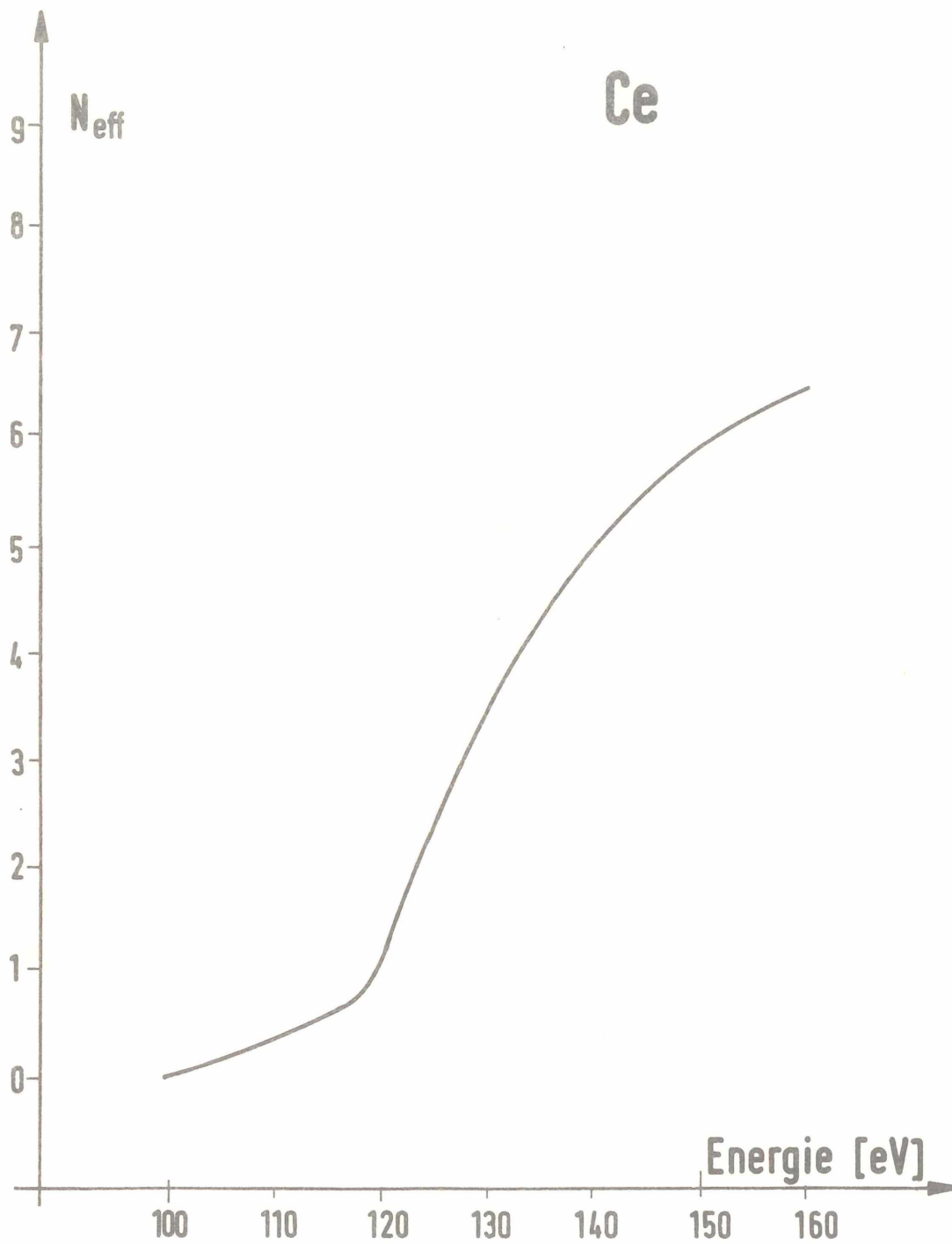
Abbildung 9a : Zahl der effektiven Elektronen (Cer)
