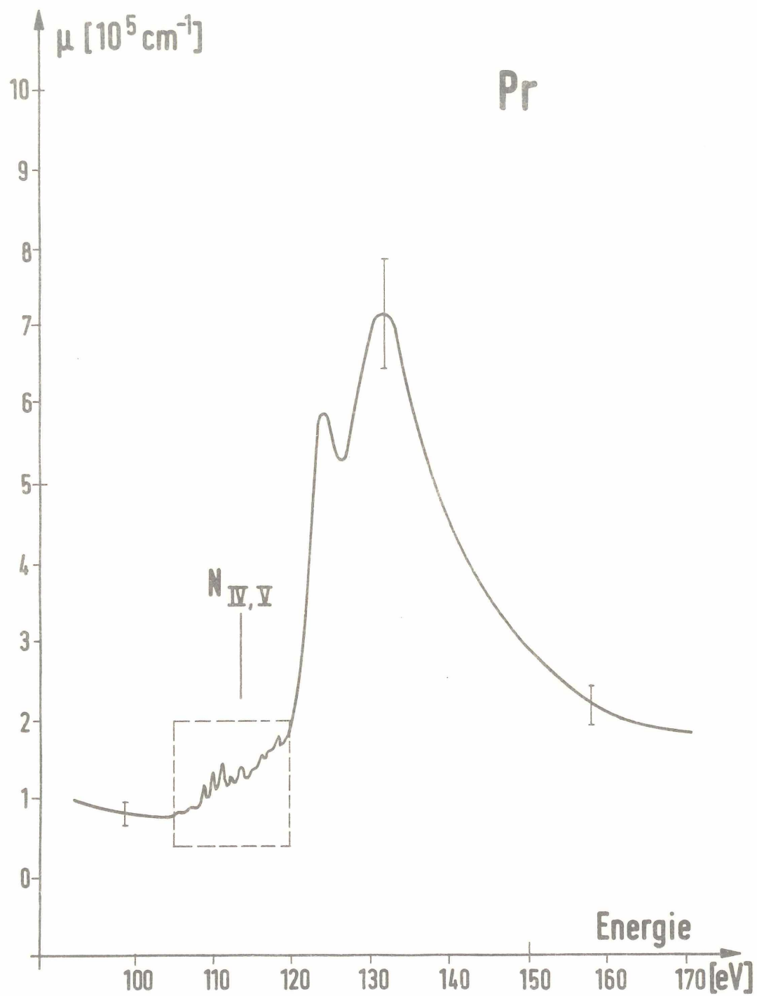
Abbildung 13 : Absorptionsspektrum von Praseodym
