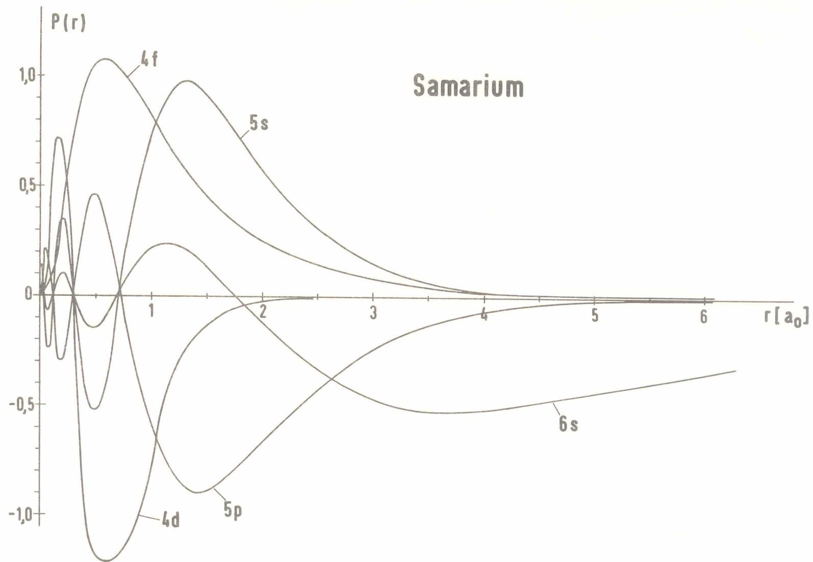
Abbildung 1 : Radiale Wellenfunktionen von Samarium
