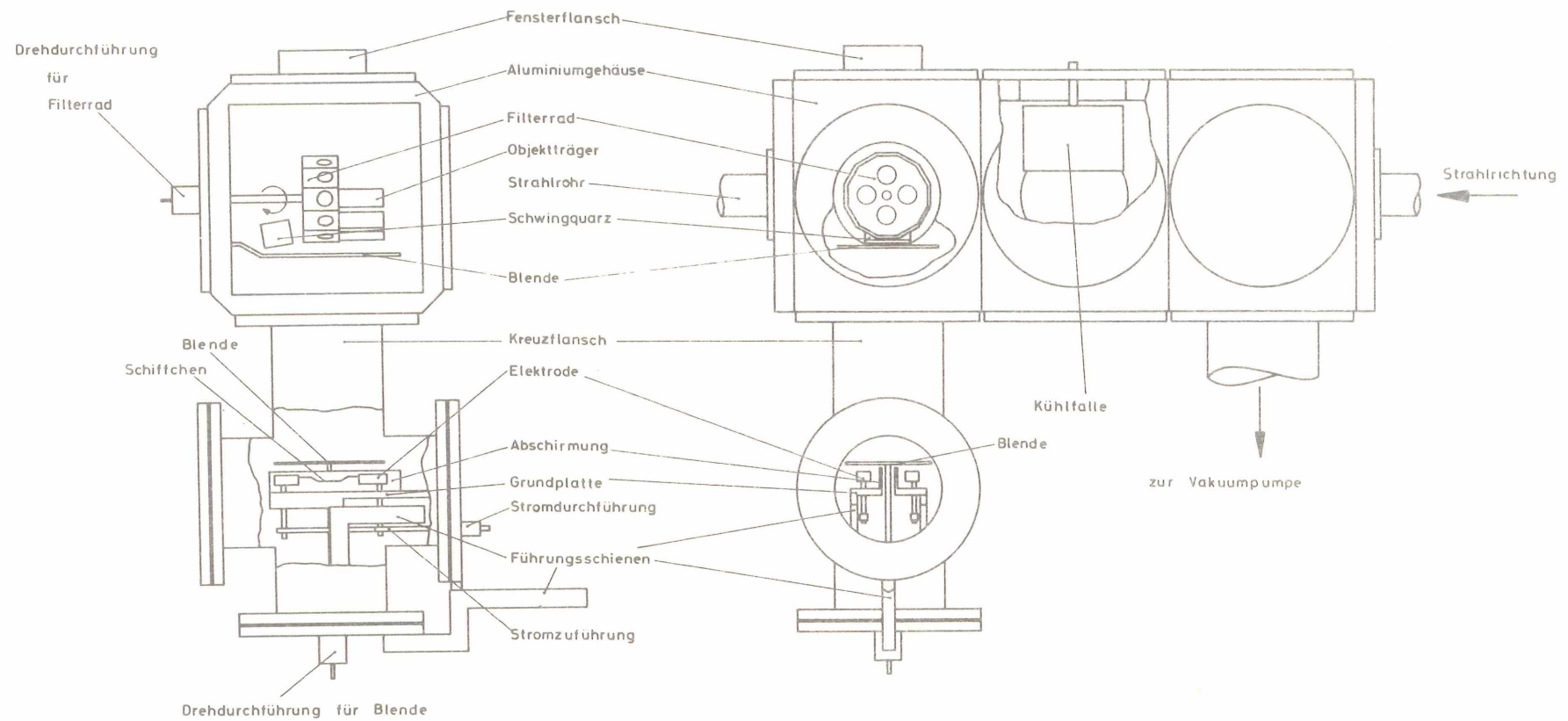
Abbildung 6 : Skizze der Aufdampfapparatur
