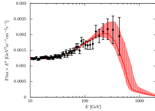
(f) L_3L_1E_2^c positron flux
