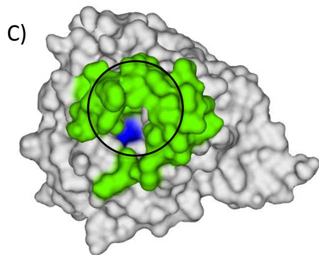
hMGL open; (PDB: 3JW8)
